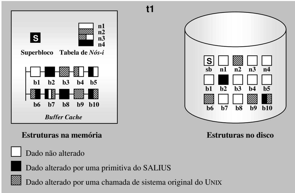
Figura 5.6: Estado de um sistema de arquivos na ocasião de um crash .
