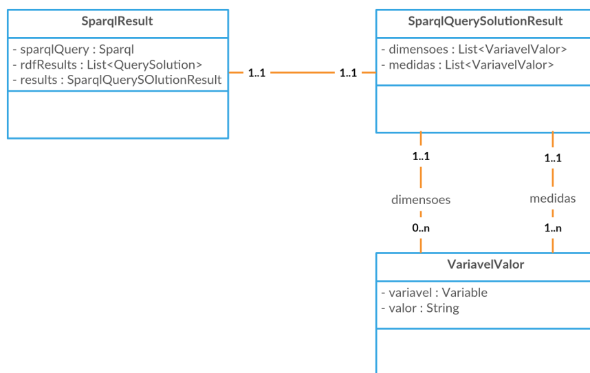
Figura 14: Diagrama de Classes para objeto SparqlResult
