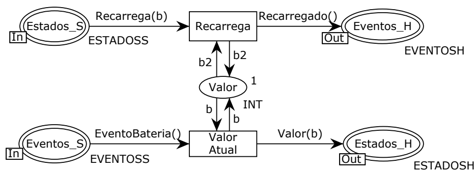
Figura 5.8: Sub-módulo da bateria do sistema.
