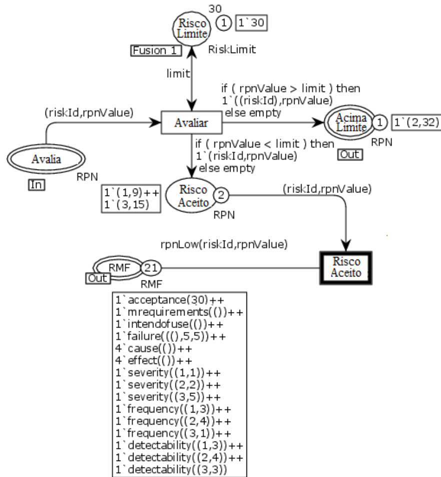
Figura 5.24: Amostra de simulação do módulo de avaliação de risco.
