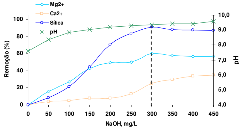
Figura 4.6 – Ponto de dosagem de NaOH
