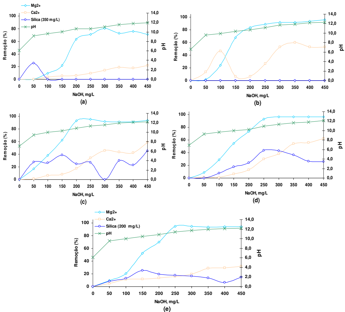
Figura 4.2 – Comportamento da variação de sílica a 350 mg/L em função da dosagem de NaOH para remoção de Mg 2+ e Ca 2+ dureza e razão molar diferentes: (a) Dureza a 50 mg/L, C_{Mg^{2+}} 4,05 mg/L, R_{Eq,g} = 0,5 ; (b) Dureza a 50 mg/L, C_{Mg^{2+}} a 8,09 mg/L, R_{Eq,g} = 2 ; (c) Dureza a 250 mg/L, C_{Mg^{2+}} a 20,32 mg/L, R_{Eq,g} = 0,5 ; (d) Dureza a 250 mg/L, C_{Mg^{2+}} a 40,5 mg/L, R_{Eq,g} = 2 ; (e) sílica a 200 mg/L dureza a 150 mg/L, C_{Mg^{2+}} a 18,21 mg/L e R_{Eq,g} = 1
