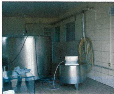
Foto3. Tanques de equilíbrio e pasteurização
