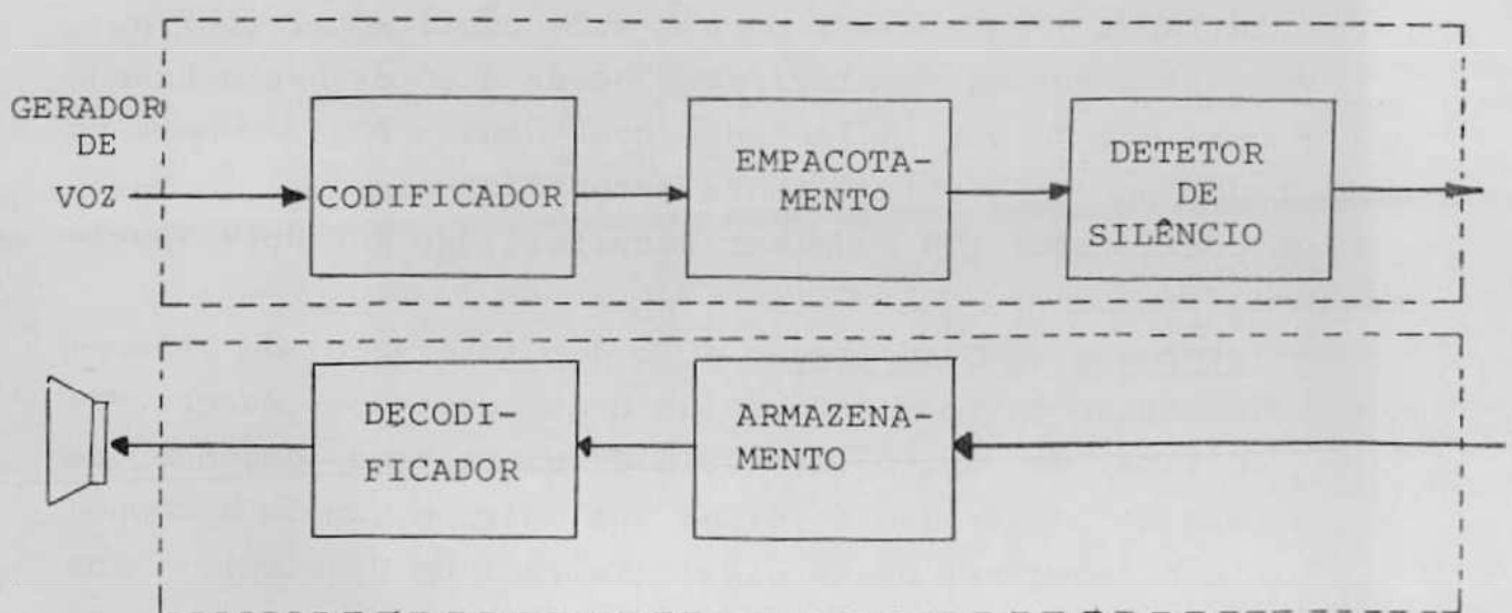
Figura 5 - Componentes básicos de uma estação de voz
