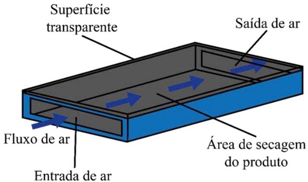
FIGURA 2 - SECADOR PASSIVO
