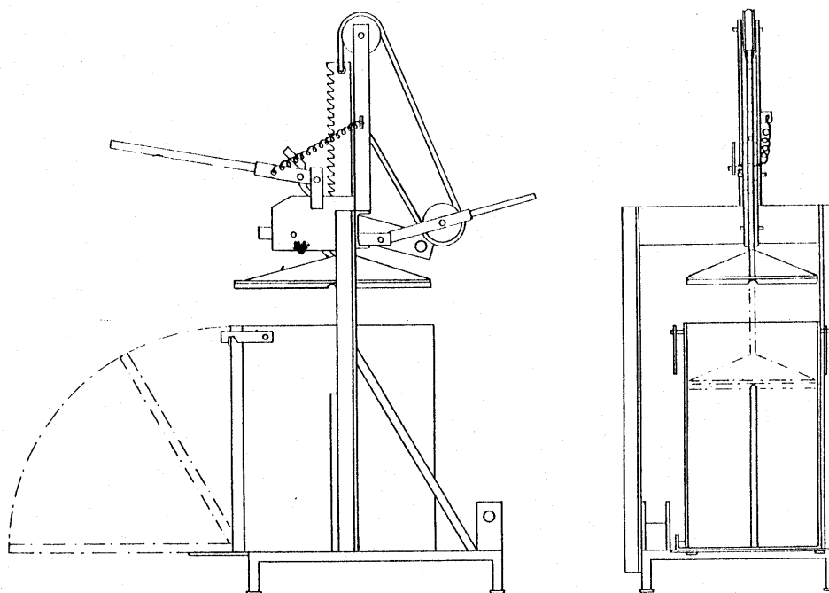
Figura 39 - Enfardadora manual
