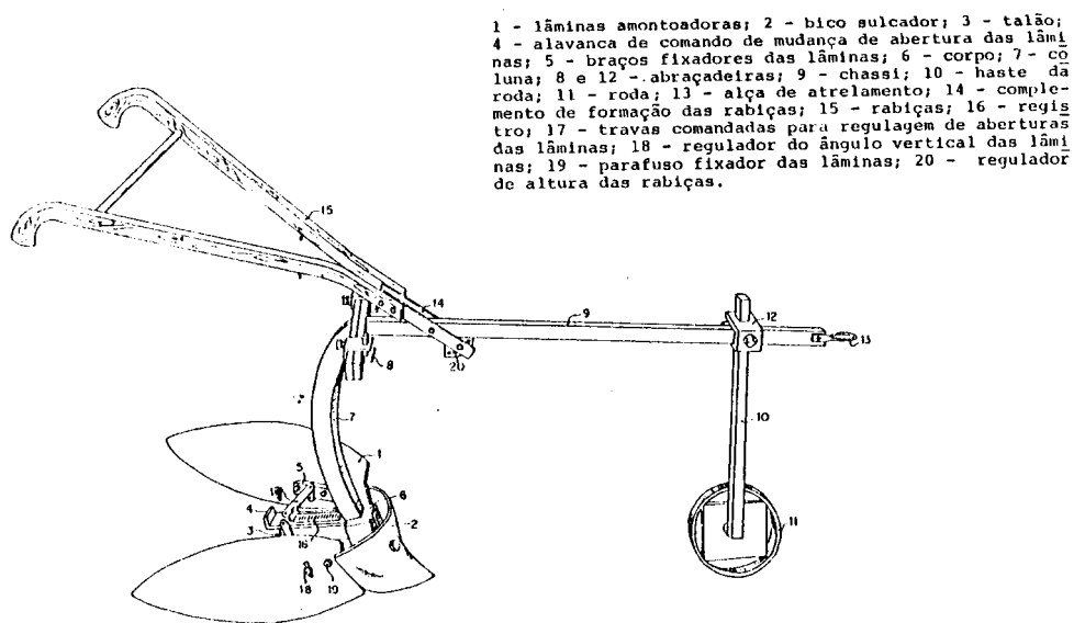
Figura 10 - Cultivador de enxadas helicoidais para “amontoa” em batateira ( solanum tuberosum L. ). Fonte: PEREIRA et al. (1986.)
