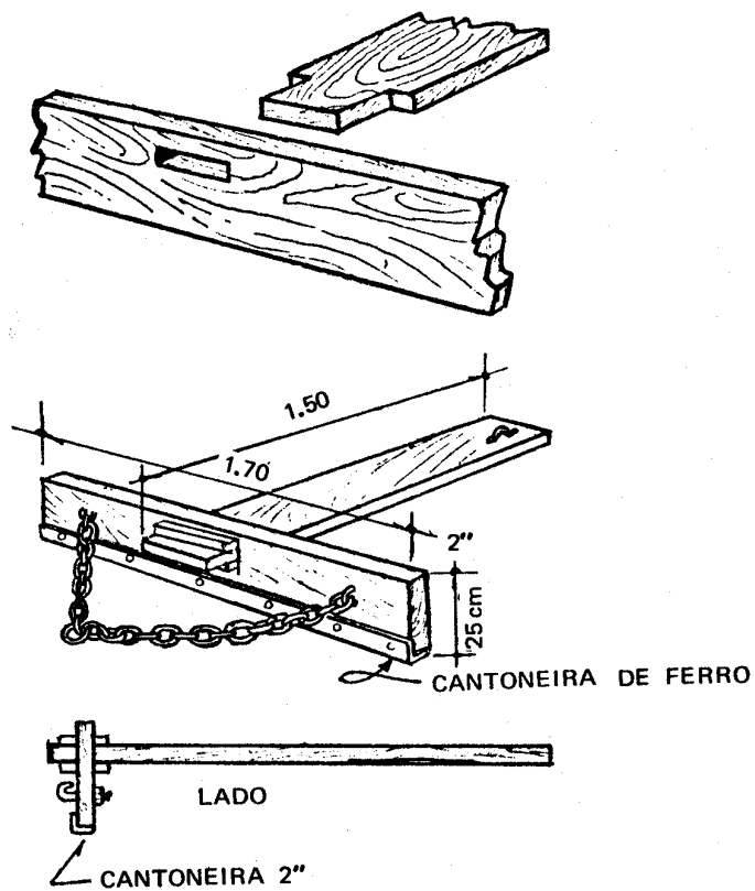
Figura 22 - Nivelador de solo
