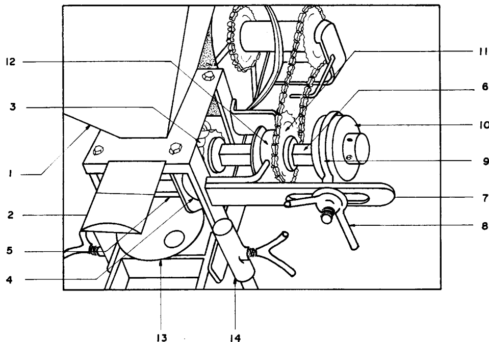
Figura 19 - Semeadora com mecanismo tipo “cilindro acanalado”.
