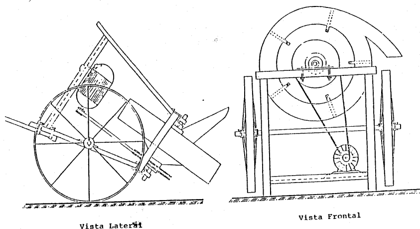
Figura 14 - Trilhadora de fluxo radial para sorgo. Fonte: SOBRINHO et al. (19..).
