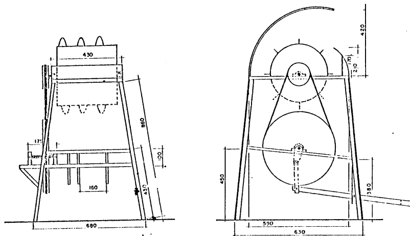
Figura 9 - Batedora mecânica de arroz Fonte: RAIOL et al. (19..)
