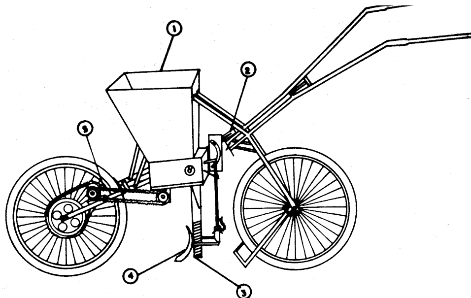
Figura 20: Adubadora com sistema tipo disco dentado
