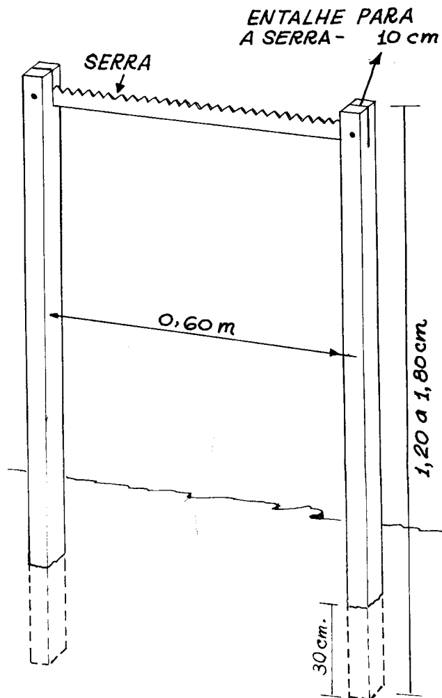
Figura 27 - Cortador de rama de mandioca.
