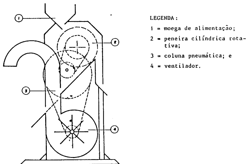
Figura 11 - Máquina de limpeza de milho, a ar, com peneira cilíndrica rotativa. Fonte: TEIXEIRA et al.
