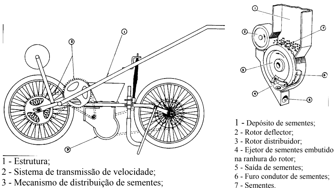
Figura 19 - Semeadora de ervilha com mecanismo tipo rotor vertical. Fonte: ROCHA (1990).
