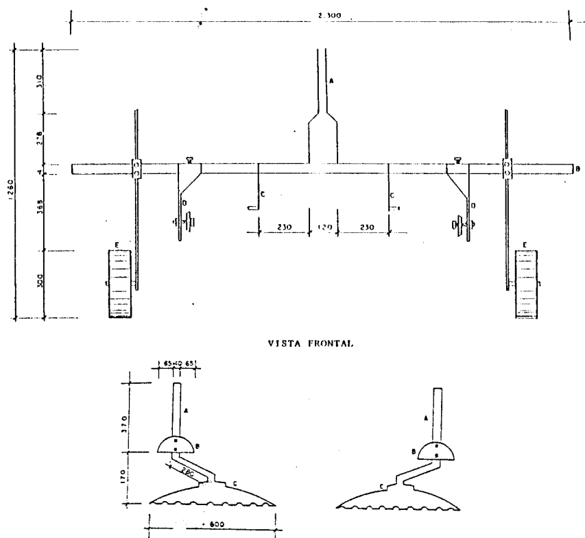
Figura 8 - Implemento para arrancar e enleirar feijão. Fonte: NAGAOKA et al. (1995.)
