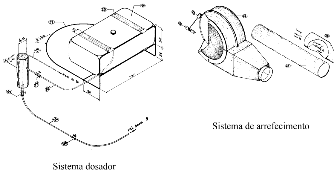
Figura 15 - Esquema dos principais componentes do Termonebulizador Adaptável à motocicleta. Fonte: CRUZ et al. (1985)
