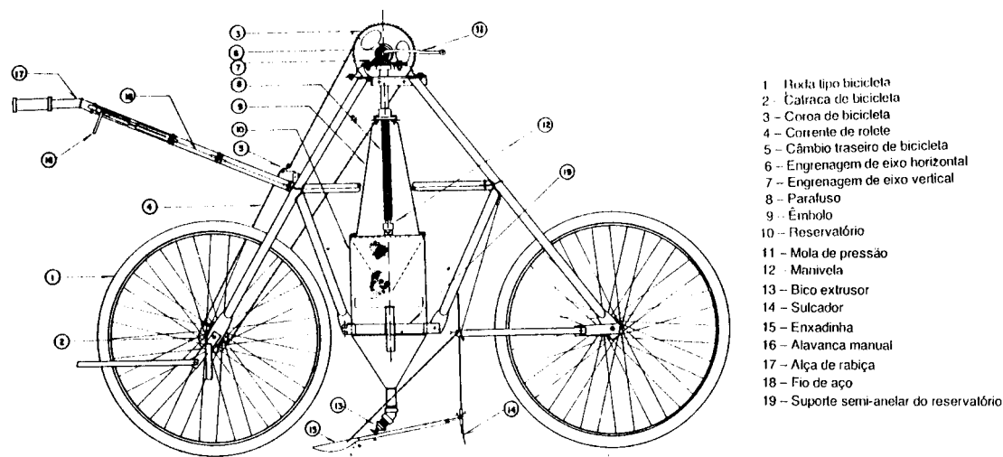
Figura 12 - Sementeira de fluido-semente montada sobre rodas.
