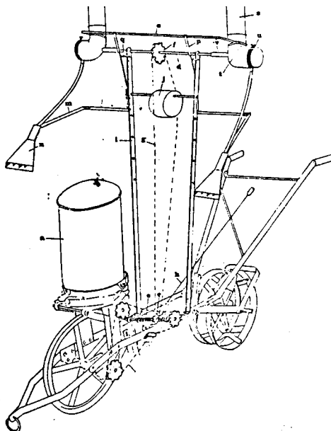
Figura 5 - Desenho esquemático do implemento para aplicação de inseticida granulado diretamente no cartucho das plantas de milho ou sorgo, adaptado à plantadeira de tração animal.
