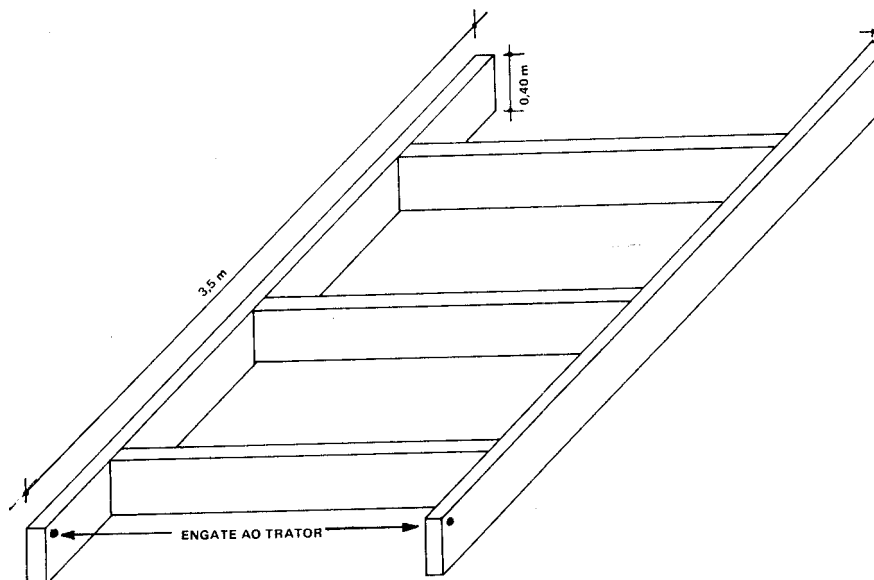
Figura 23 - Nivelador de solo em formato de escada.
