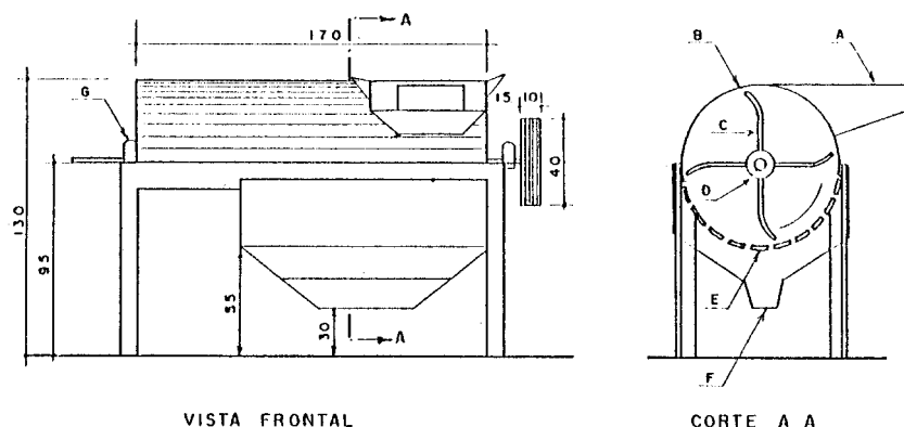
Figura 13 - Trilhadora de feijão.
