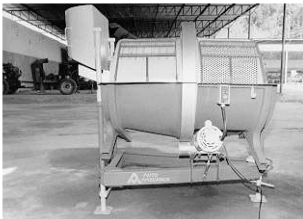
Figura 7 - Classificadora Rotativa de Sementes de Milho. Fonte: BERTAUX & SCHAUM.
