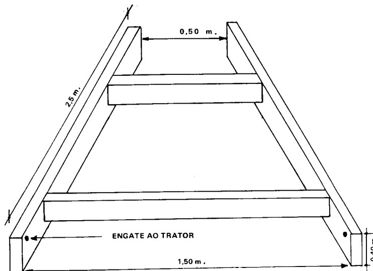
Figura 25 - Enleirador de madeira.
