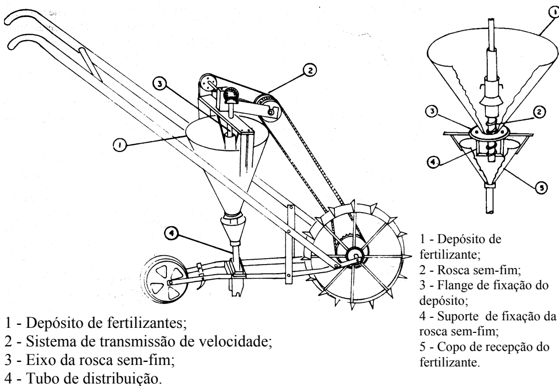
Figura 21. Adubadora com sistema tipo rosca sem-fim vertical.
