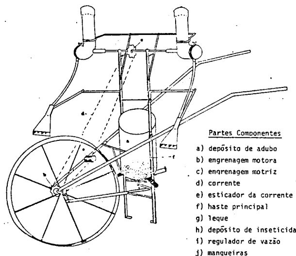
Figura 6 - Desenho esquemático do implemento para aplicação de inseticida granulado diretamente no cartucho das plantas de milho ou sorgo, adaptado a adubadeira manual Fonte: Finch et al (1982).
