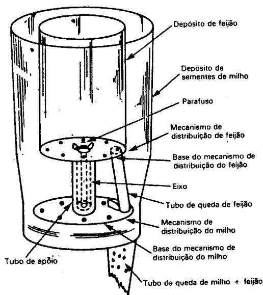
Figura 1 - Dispositivo para semeadura simultânea de milho e feijão.
