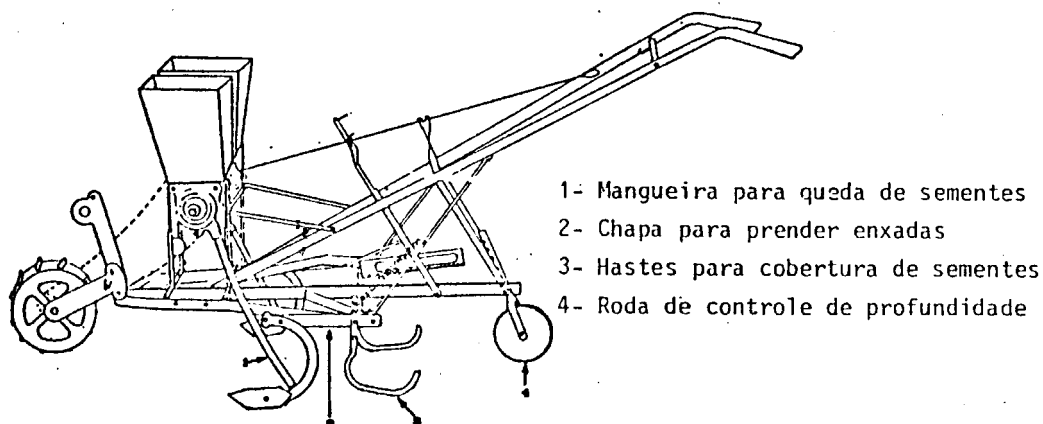
Figura 2 - Semeadora desenvolvida pelo CNPMS-ENBRAPA, que permite a semeadura simultânea de duas linhas de feijão após a maturação fisiológica do milho.
