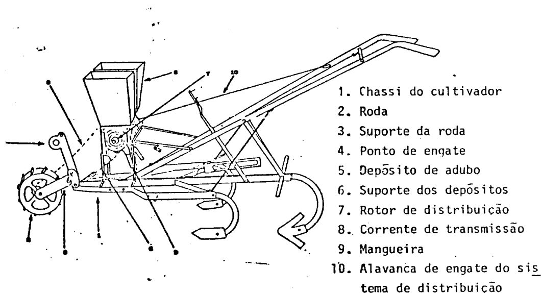
Figura 3 - Cultivador-Adubadora desenvolvido pelo CNPMS-EMBRAPA, que permite a adubação em cobertura, incorporação e cultivo simultaneamente.
