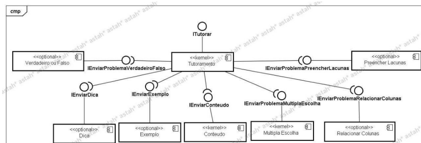
Figura 4.12: Exemplo de Configuração arquitetural na camada de sistema
