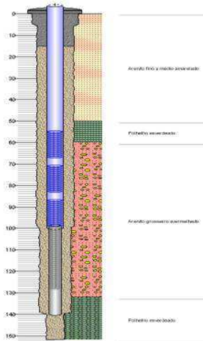
Quadro 11 – Dados litológicos PT 4
