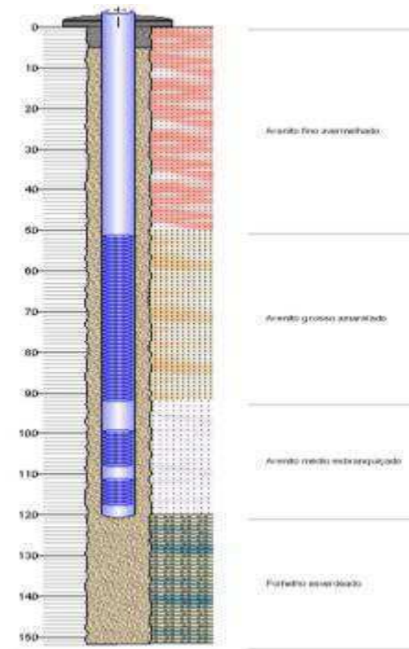
Quadro 14 – Dados litológicos PT 27
