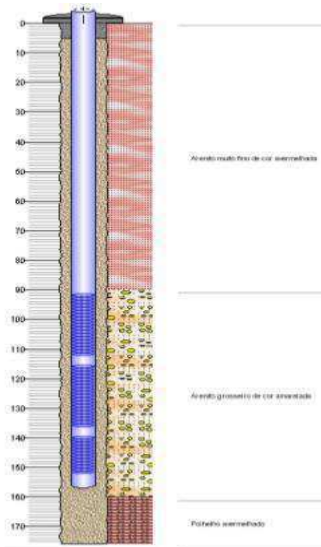
Quadro 12 – Dados litológicos PT 30
