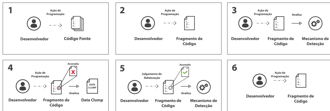
Figura 6.2: Etapas da Detecção Interativa.
