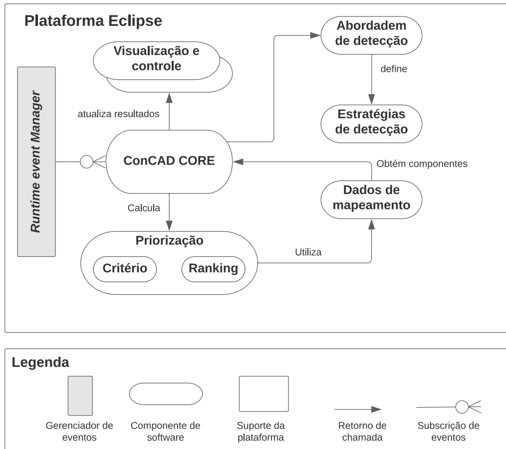
Figura D.1: Arquitetura da Ferramenta Eclipse ConCAD .
