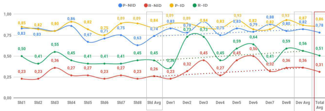
Figura 7.4: Resultados em Termos de Precision e Recall .
