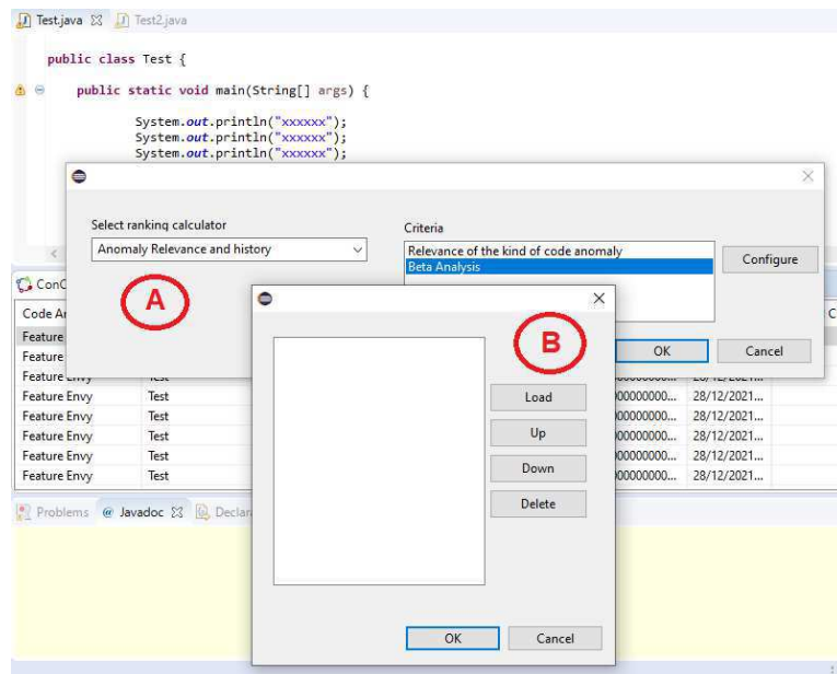
Figura D.6: Priorização Baseada no Histórico.
