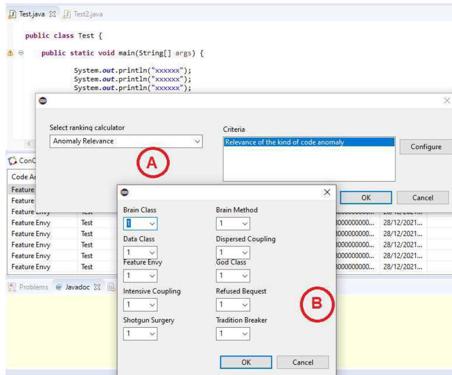
Figura D.4: Priorização por Tipo de Anomalia.
