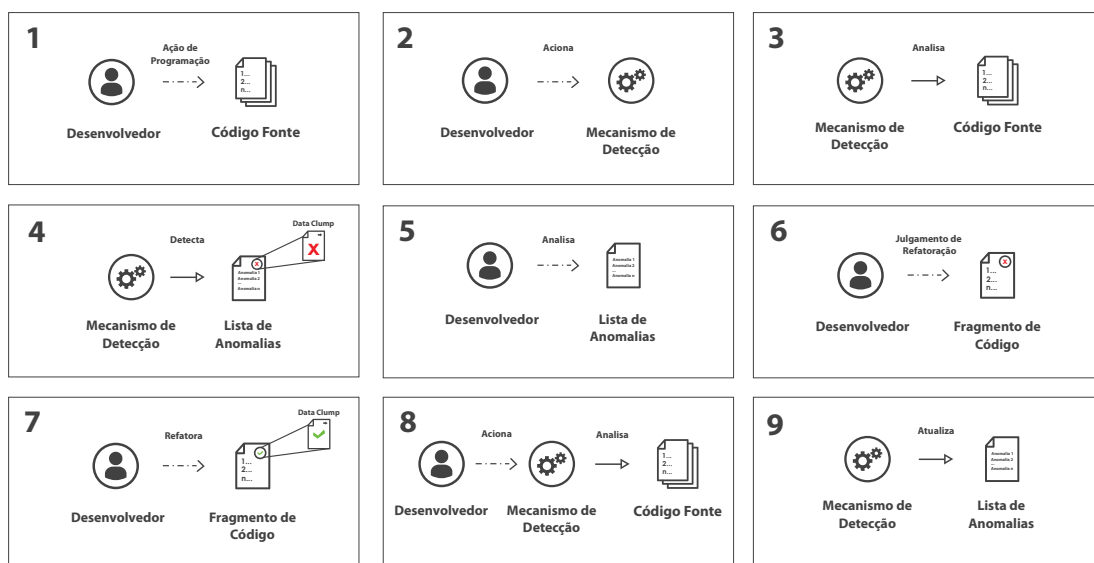
Figura 2.2: Etapas da Detecção Não-Interativa.
