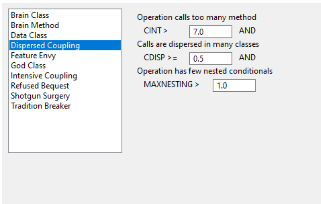
Figura B.4: Estratégia de Detecção - Dispersed Coupling .
