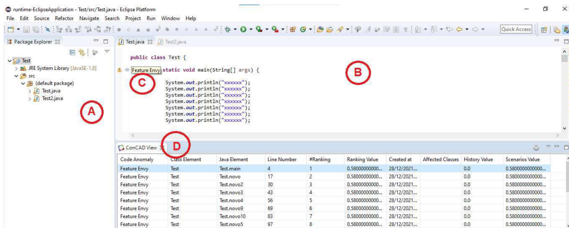
Figura D.2: Visão Geral da Ferramenta Eclipse ConCAD .
