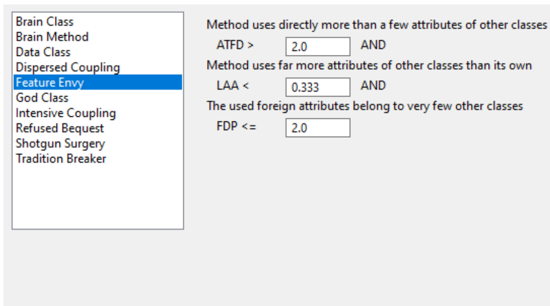
Figura B.5: Estratégia de Detecção - Feature Envy .
