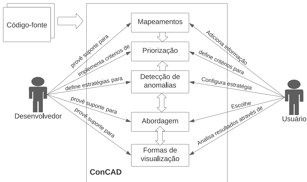
Figura 7.1: Fluxo de Trabalho da Ferramenta Eclipse ConCAD .
