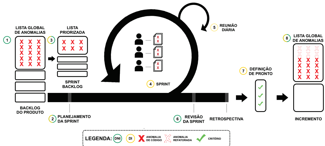
Figura 9.2: Etapas de Integração da Abordagem DI no Arcabouço do Scrum .
