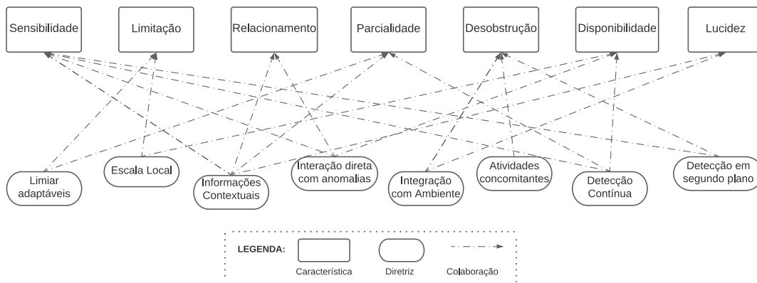
Figura 6.3: Mapeamento das Características e Diretrizes.
