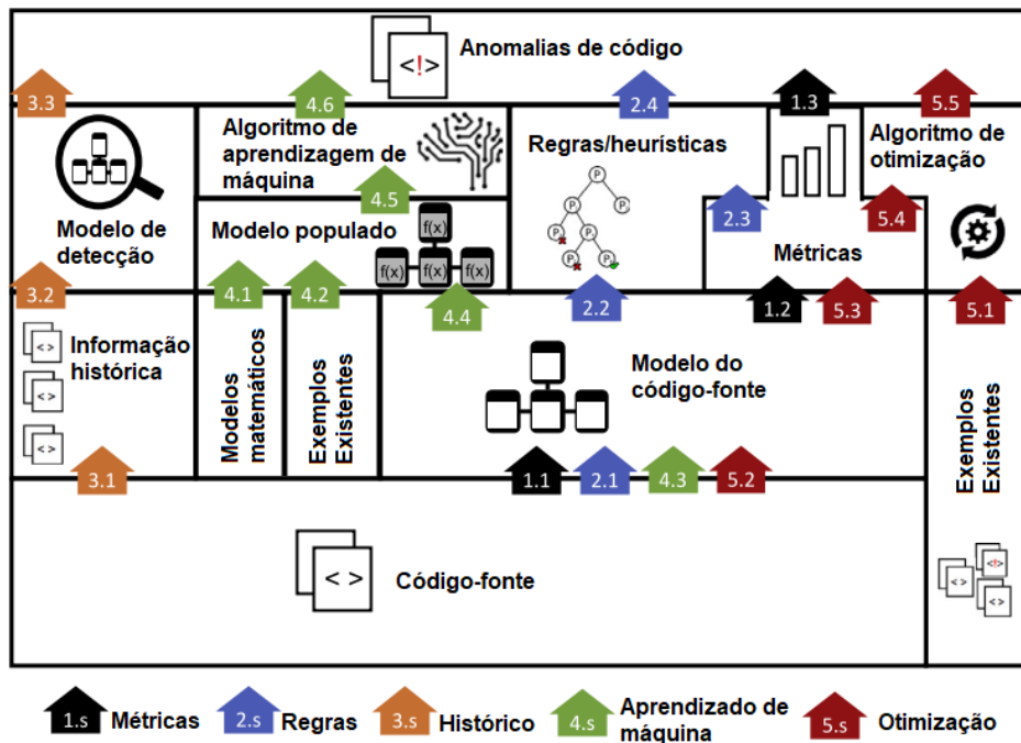
Figura 5.2: Visão em Camadas dos Métodos de Detecção.
