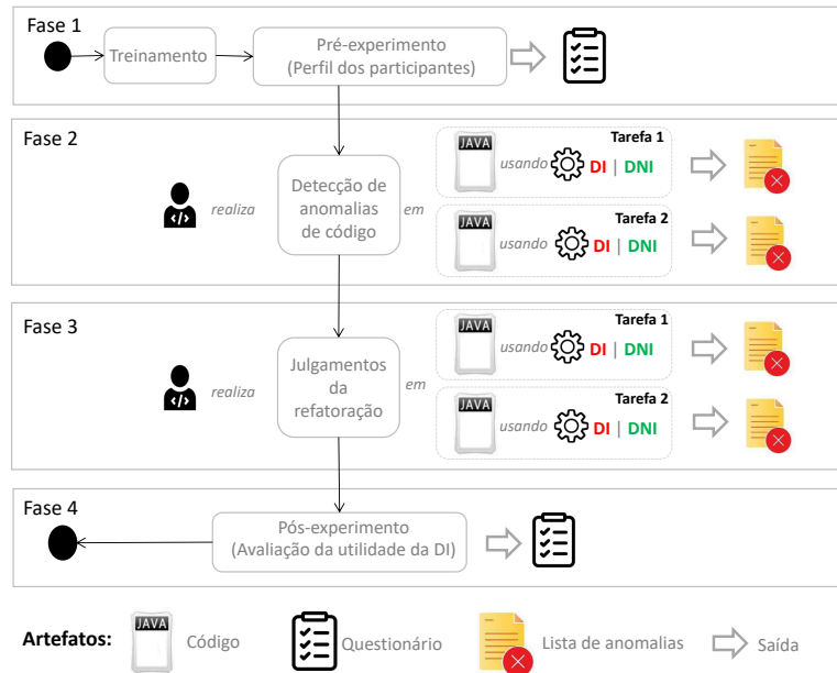
Figura 7.3: Etapas de Execução do Experimento.
