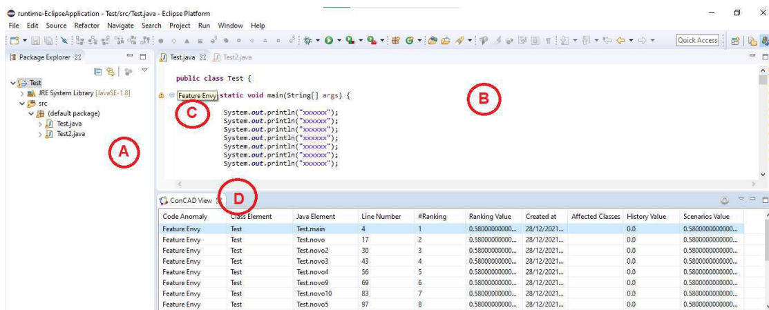
Figura 7.2: Visão Geral da Ferramenta Eclipse ConCAD .
