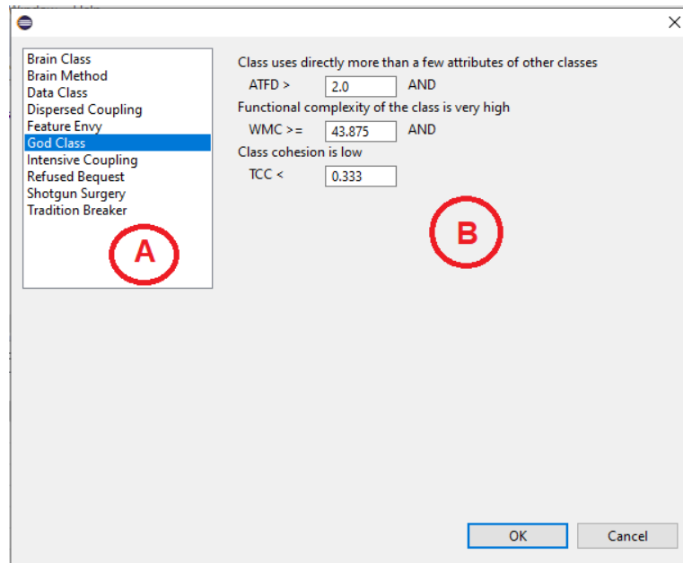
Figura D.3: Definição da Estratégia de Detecção.
