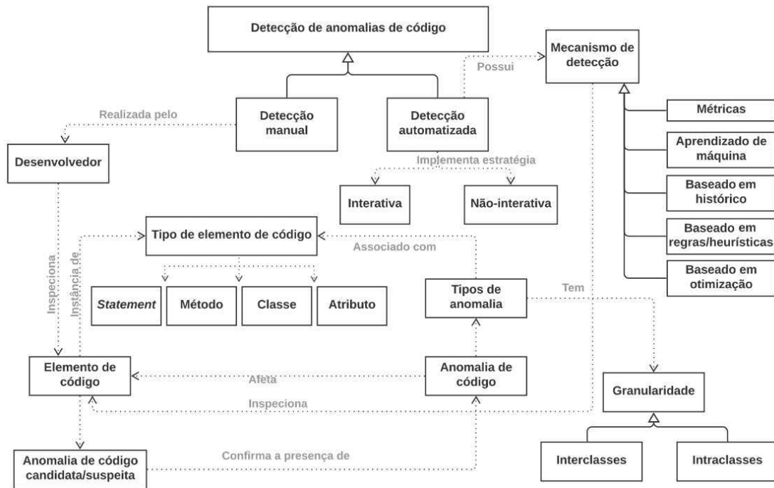
Figura 2.1: Conceitos da Detecção de Anomalias.
