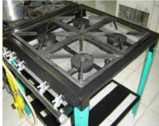
FIGURA 34 | Fogão utilizando a energia térmica proveniente da queima do biogás
