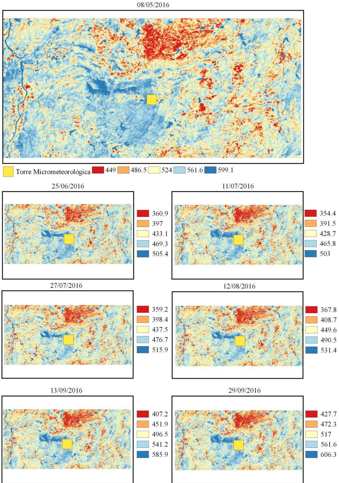
Figura 18. Mapas temáticos do saldo de radiação instantâneo ( \text{Wm}^{-2} ) dos produtos do OLI/TIRS Landsat 8 na Torre Micrometeorológica referentes aos dias selecionados para a pesquisa em 2016 (Projeção: geográfica, Datum: WGS 84).
