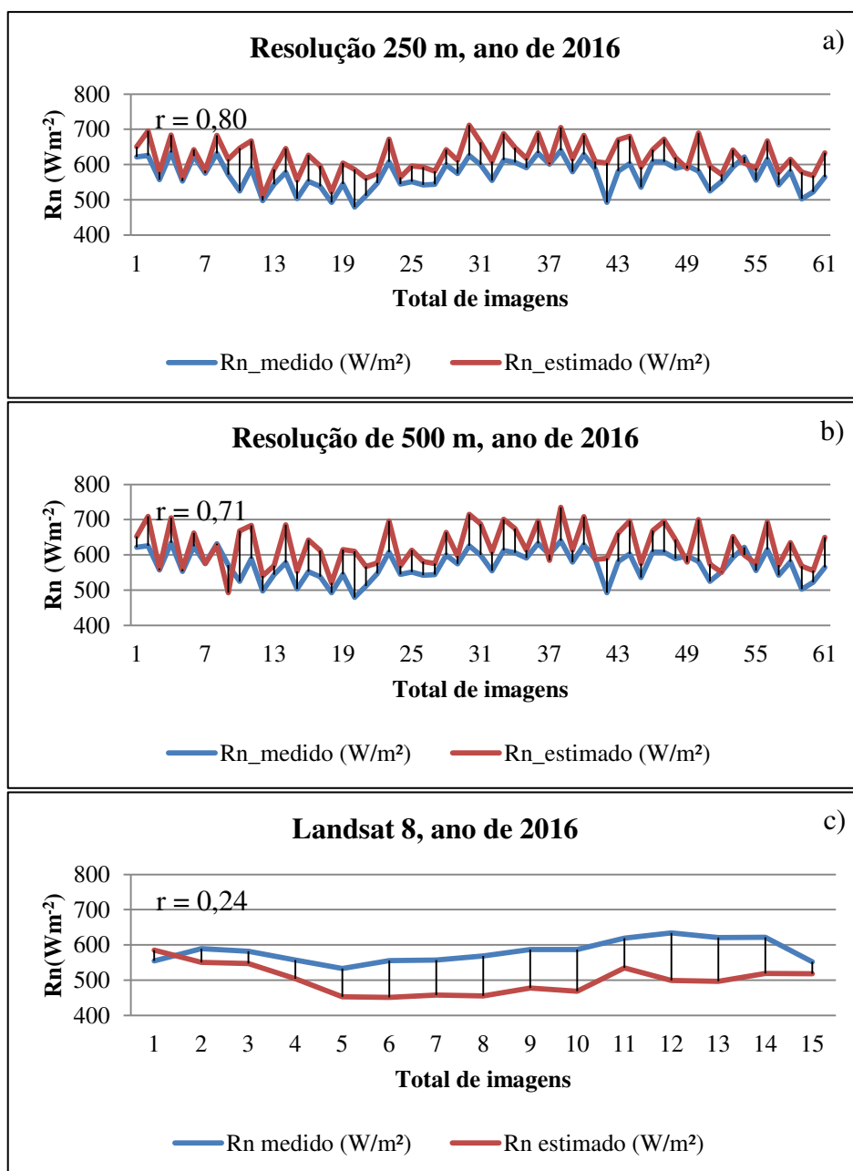
Figura 22. Representação gráfica dos valores de R_n instantâneo estimado e medido para os dias em estudo no ano de 2016 para os produtos: a) MODIS, resolução de 250 m; b) MODIS, resolução de 500 m e c) OLI/TIRS Landsat 8.
