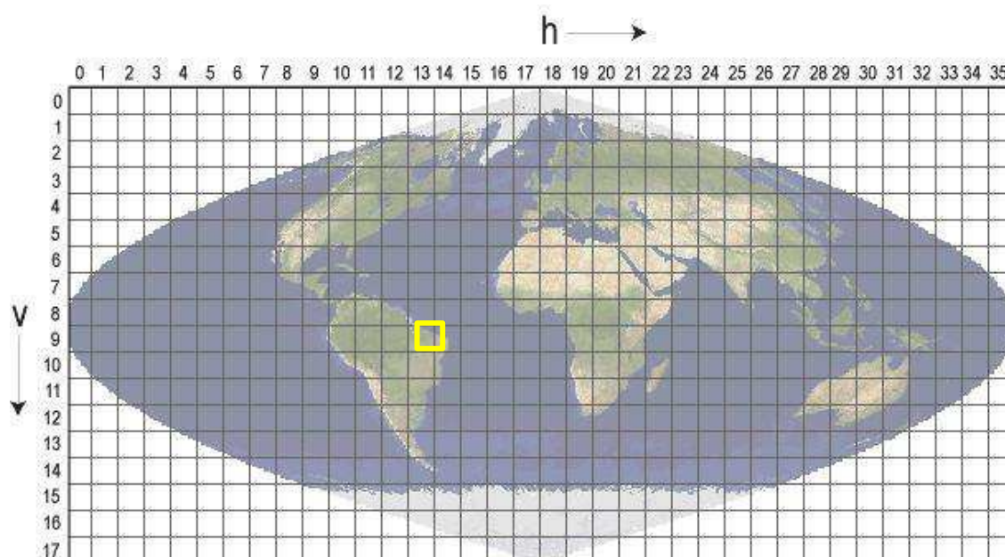
Figura 6. Tiles do sensor MODIS, com destaque para o tile em que se encontra a área de estudo (Fonte: NASA, 2017).
