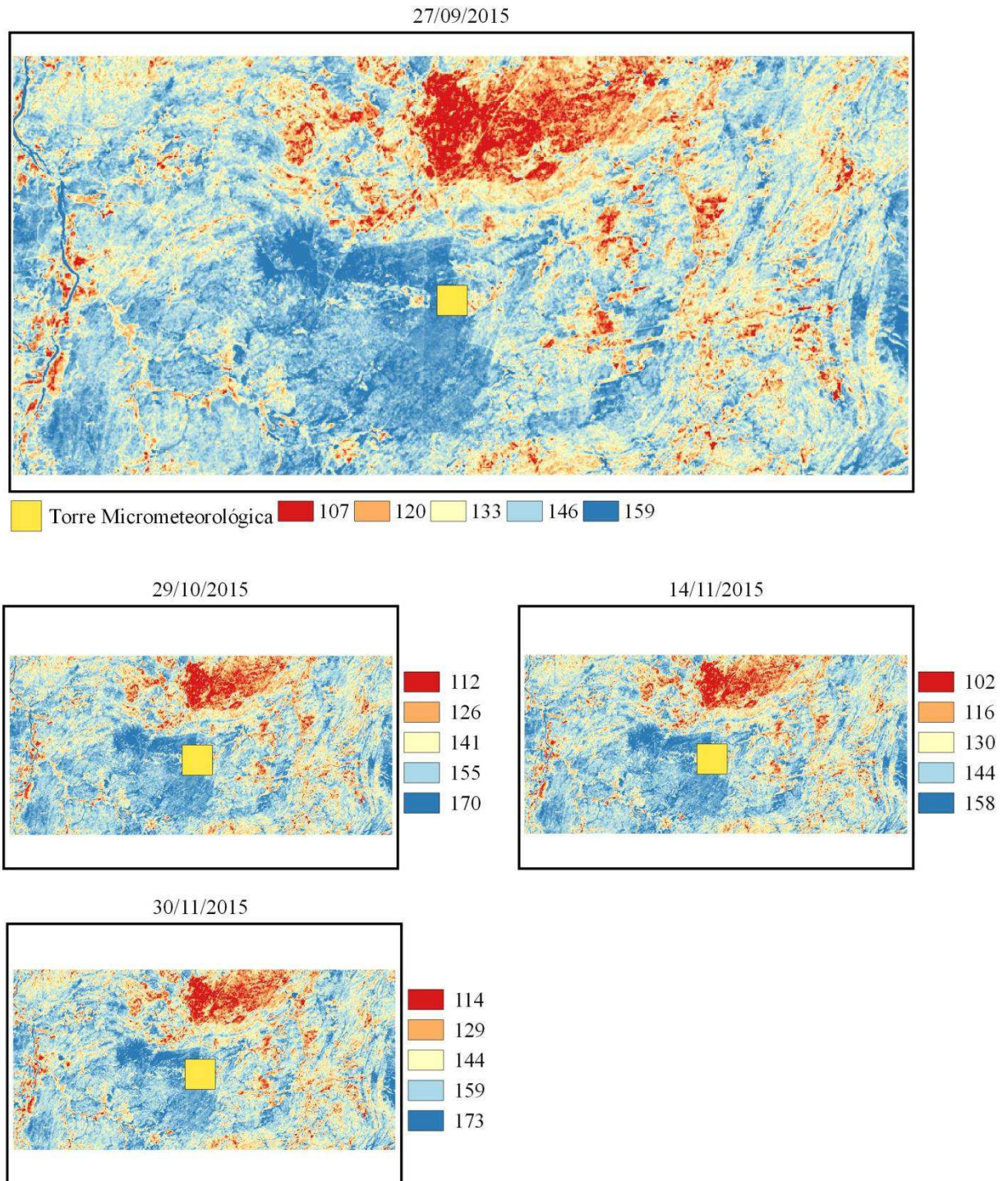
Figura 23. Mapas temáticos do saldo de radiação diário ( Wm^{-2} ) dos produtos do OLI/TIRS Landsat 8 na Torre Micrometeorológica referentes aos dias selecionados para a pesquisa em 2015 (Projeção: geográfica, Datum: WGS 84).
