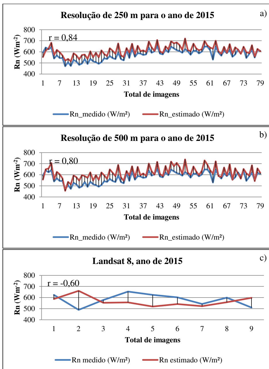
Figura 21. Representação gráfica dos valores de R_n estimado e medido para os dias em estudo no ano de 2015 para os produtos: a) MODIS, resolução de 250 m; b) MODIS, resolução de 500 m e c) OLI/TIRS Landsat 8.
