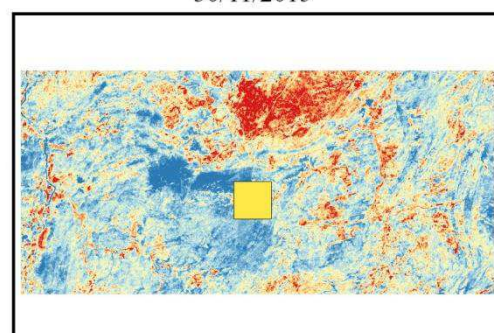
Figura 16. Mapas temáticos do saldo de radiação instantâneo obtidos com o OLI/TIRS Landsat 8 na Torre Micrometeorológica referentes aos dias selecionados para a pesquisa em 2015 (Projeção: geográfica, Datum: WGS 84).
