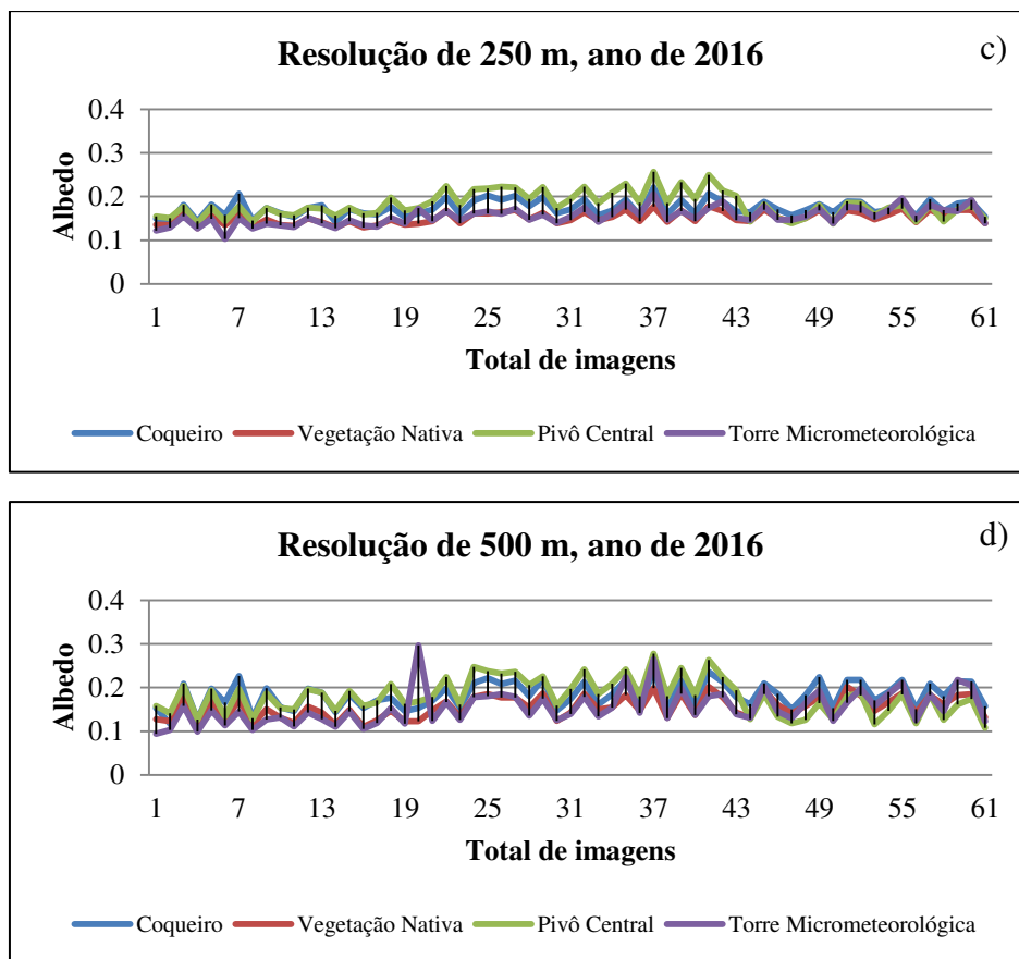
Figura 15. Comportamento do albedo de superfície dos produtos MODIS referente aos dias e alvos selecionados para a pesquisa: a) resolução de 250 m ano de 2015; b) resolução de 500 m ano de 2015; c) resolução de 250 m ano de 2016; d) resolução de 500 m ano de 2016.
