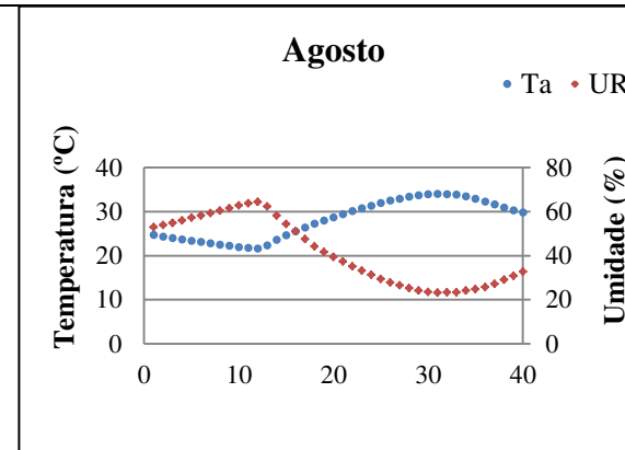
Figura 10. Ciclo médio mensal das variáveis meteorológicas, temperatura do ar - Ta (°C) e umidade relativa do ar - UR (%), para o ano de 2016
