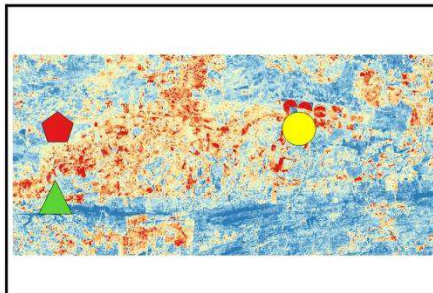
Figura 24. Mapas temáticos do saldo de radiação diário ( Wm^{-2} ) dos produtos do OLI/TIRS Landsat 8 no Perímetro Irrigado de São Gonçalo referentes aos dias selecionados para a pesquisa em 2015 (Projeção: geográfica, Datum: WGS 84).
