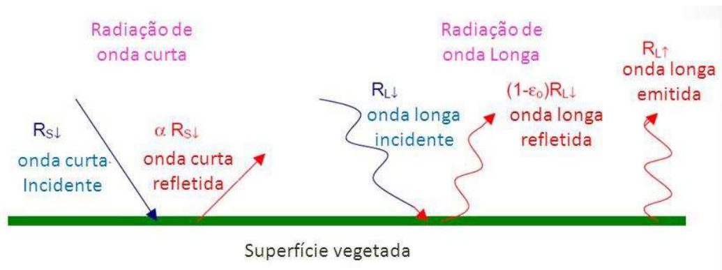
Figura 3. Representação esquemática do saldo de radiação (Adaptado de Allen, 2002).
