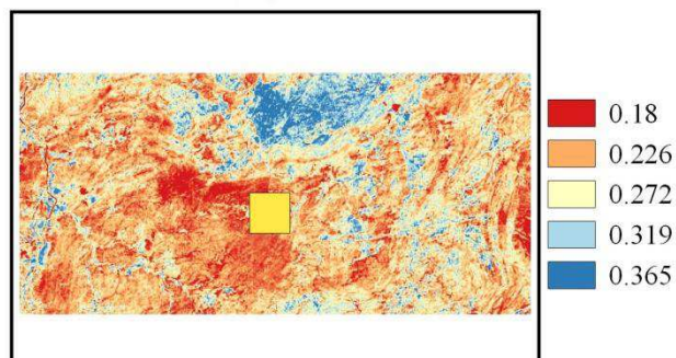
Figura 11. Mapas temáticos do albedo de superfície dos produtos do OLI-Landsat 8 na Torre Micrometeorológica referentes aos dias selecionados para a pesquisa em 2015 (Projeção: geográfica, Datum: WGS 84).
