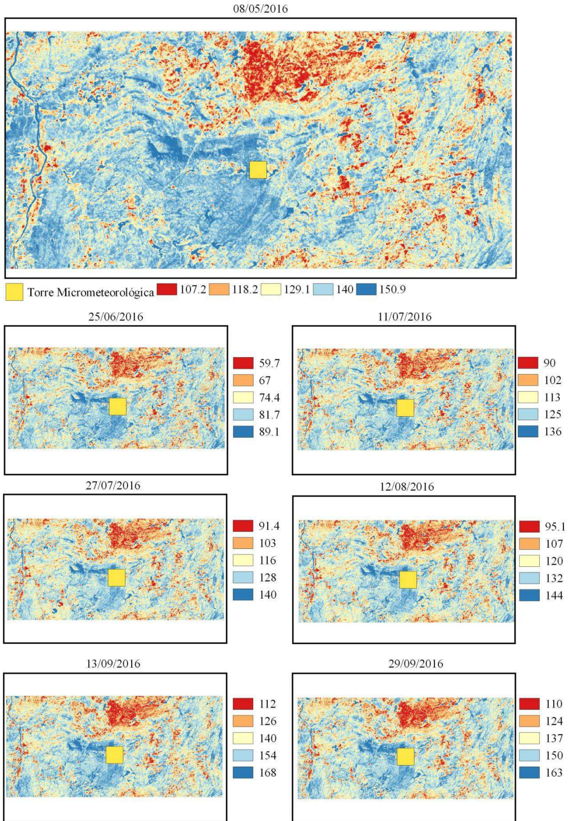
Figura 25. Mapas temáticos do saldo de radiação diário ( Wm^{-2} ) dos produtos do OLI/TIRS Landsat 8 na Torre Micrometeorológica referentes aos dias selecionados para a pesquisa em 2016 (Projeção: geográfica, Datum: WGS 84).
