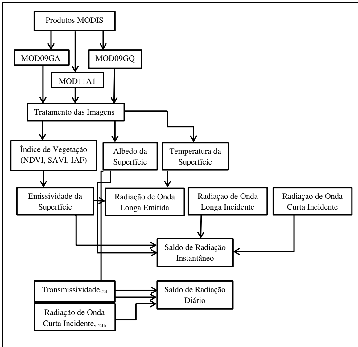
Figura 8. Etapas do processamento de obtenção do saldo de radiação à superfície – R_n , para os produtos MODIS.
