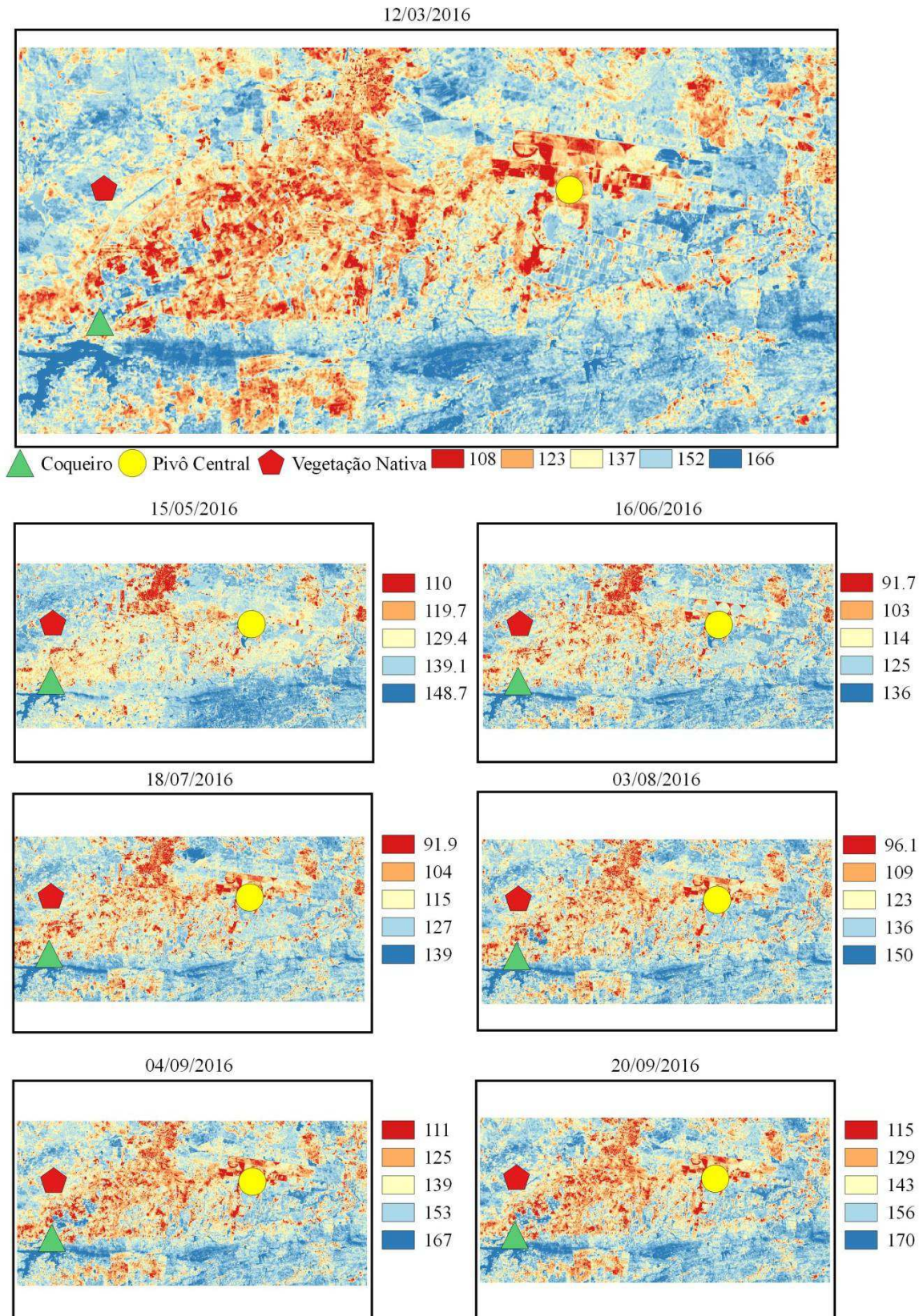
Figura 26. Mapas temáticos do saldo de radiação diário ( Wm^{-2} ) dos produtos do OLI/TIRS Landsat 8 no Perímetro Irrigado de São Gonçalo referentes aos dias selecionados para a pesquisa em 2016 (Projeção: geográfica, Datum: WGS 84).
