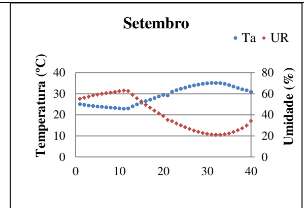
Figura 10. Ciclo médio mensal das variáveis meteorológicas, temperatura do ar - Ta (°C) e umidade relativa do ar - UR (%), para o ano de 2016
