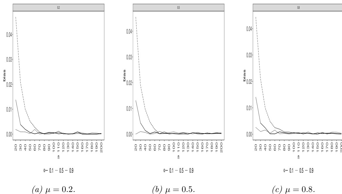
Figura 3.7: Viés de \hat{\alpha} para diferentes valores de n, \mu e \alpha de uma LBUA.
