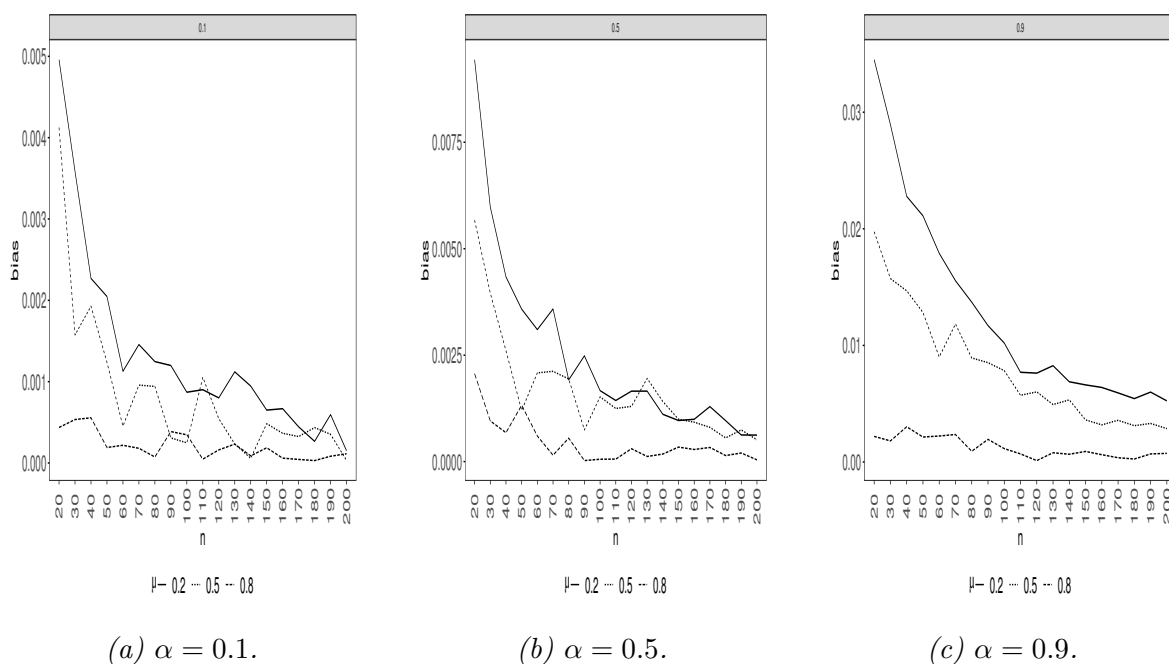
Figura 3.1: Viés de \hat{\mu} para diferentes valores de n , \mu e \alpha de uma LBZA.
