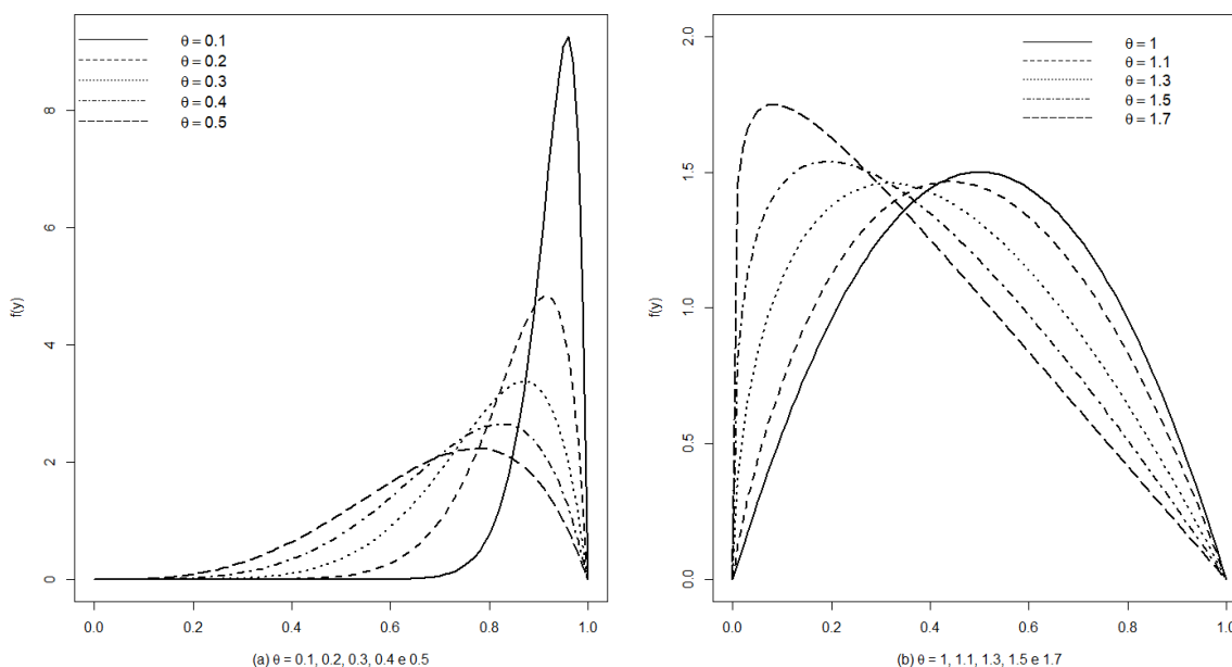
Figura 2.1: FDP de uma log-Bilal para diferentes valores de \theta
