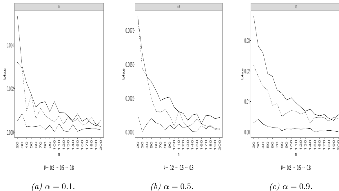
Figura 3.3: Viés de \hat{\mu} para diferentes valores de n , \mu e \alpha de uma LBUA.
