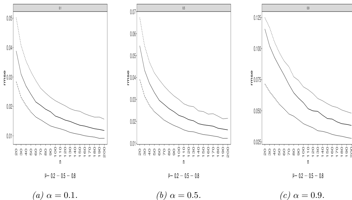
Figura 3.2: REQM de \hat{\mu} para diferentes valores de n, \mu e \alpha de uma LBZA.
