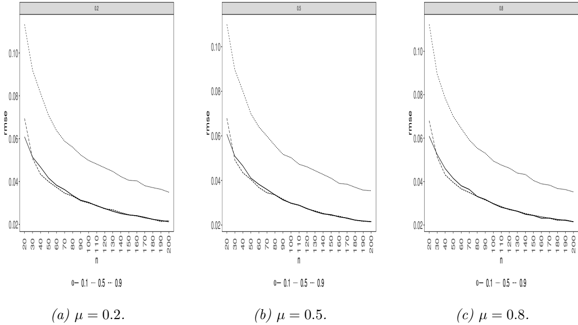
Figura 3.8: REQM de \hat{\alpha} para diferentes valores de n , \mu e \alpha de uma LBUA.
