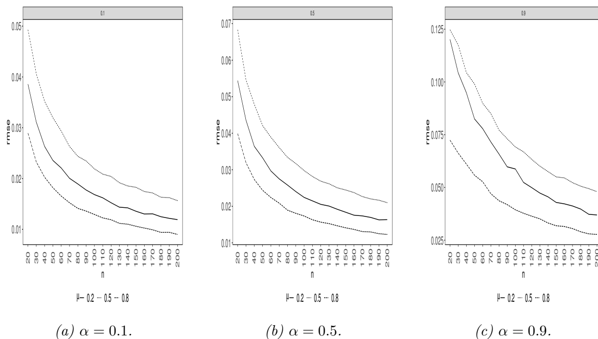
Figura 3.4: REQM de \hat{\mu} para diferentes valores de n , \mu e \alpha de uma LBUA.
