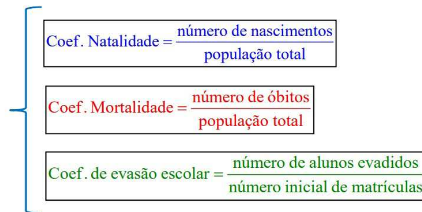
FIGURA 3 – FÓRMULAS PARA O CÁLCULO DE COEFICIENTES
