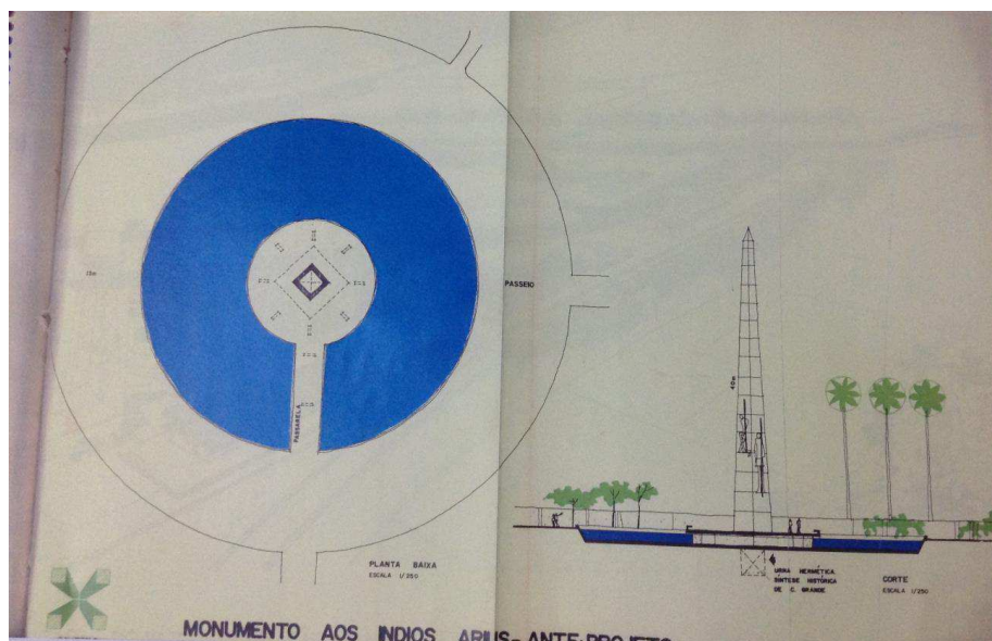
Figura 22: Planta do Obelisco do Parque do Açude Novo (PTA)
