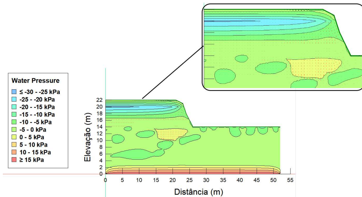
Figura 50-Infiltração no quinto dia pós-evento de chuva com 24h e 72h de duração e precipitação antecedente do talude João Lourenço
