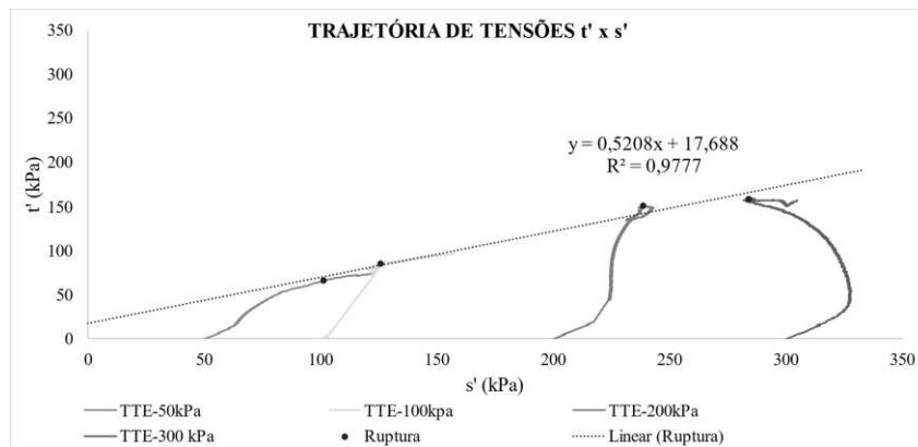
Figura 45-Trajetoórias de tensão efetiva para os espaços s'x t' para os solos MMB, MMC e MMT
