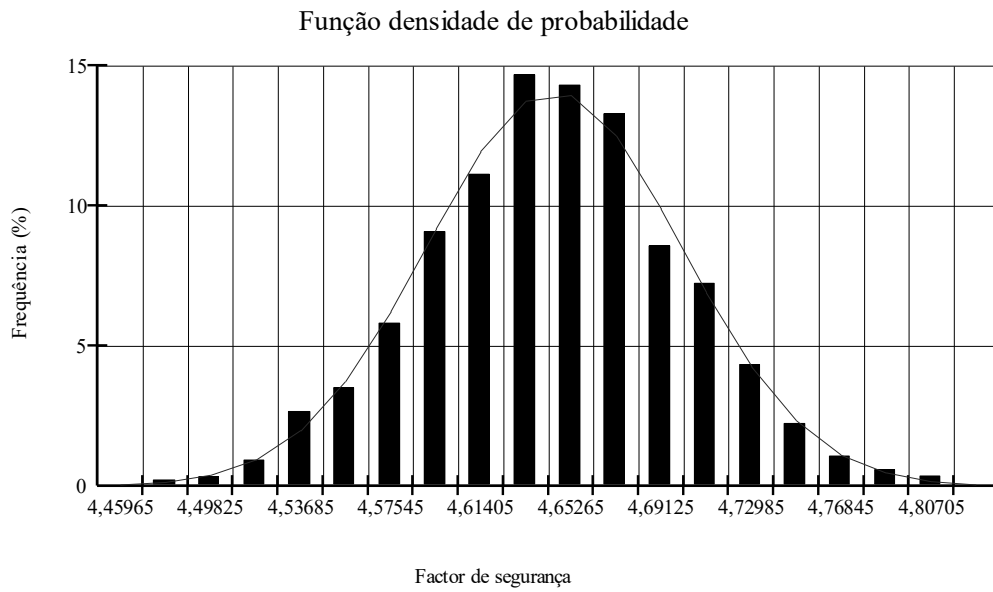
Figura 81-Distribuição de probabilidade do talude MM para 2mm/h durante 24h sem precipitação antecedente
