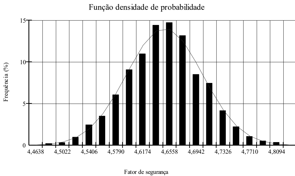
Figura 82-Distribuição de probabilidade do talude MM para 2mm/h durante 72h sem precipitação antecedente
