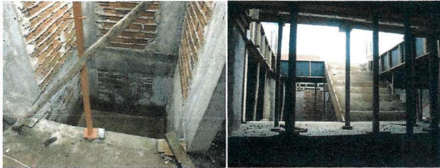
Figura 10 e Figura 11 – Fechamento de alvenaria do poço do elevador e escada.
