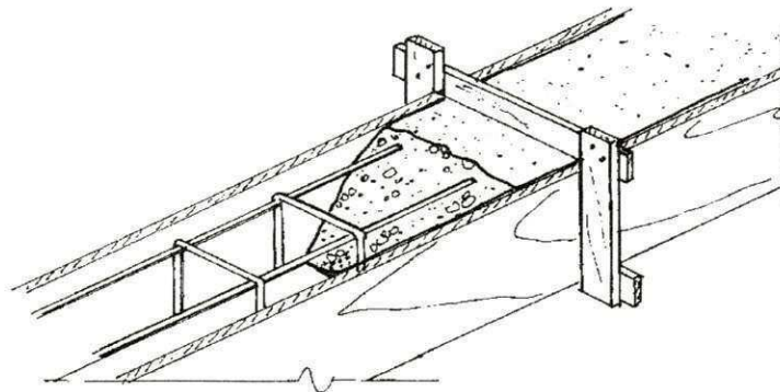
Figura 12. Concretagem de viga
