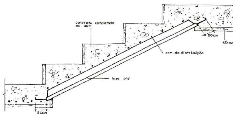
Figura 40. Corte da escada
