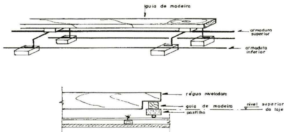
Figura 14. Passarela para movimentação sobre laje
