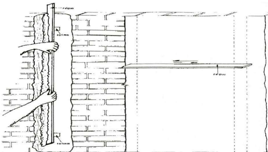
Figura 27. Nivelamento da argamassa
