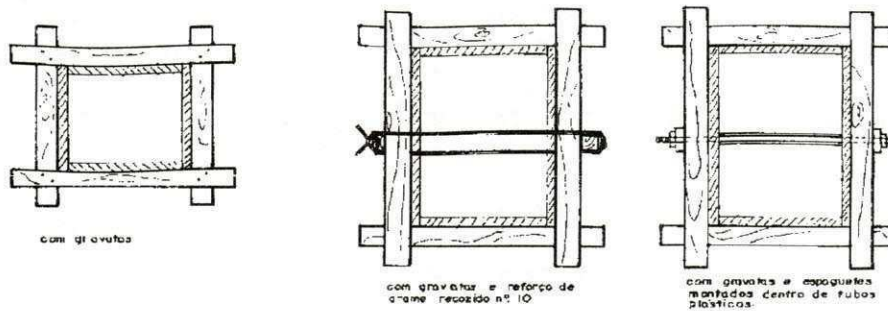
Figura 5. Seção das gravatas mais usuais para pilares
