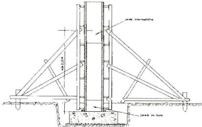
Figura 4. Escoramento de madeira para pilar
