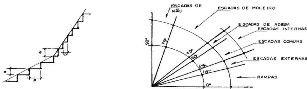
Figura 36. Mudança de Inclinação das escadas
