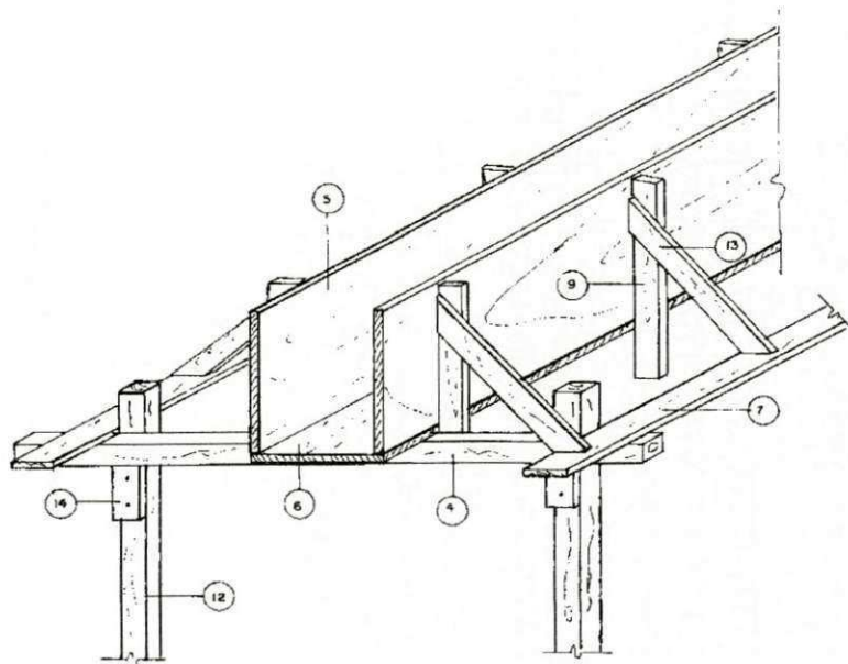
Figura 9. Outro tipo de fôrma e escoramentos de vigas
