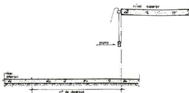
Figura 37. Execução da escada
