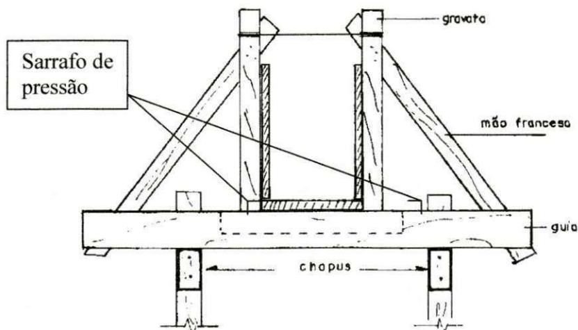
Figura 8. Fôrma e escoramentos de vigas
