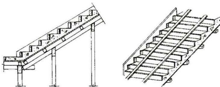
Figura 39. Fôrmas para escada
