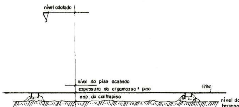
Figura 30. Nivelamento para piso
