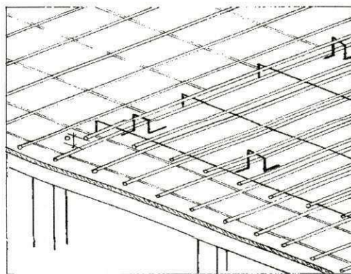
Figura 13. Distância entre armaduras
