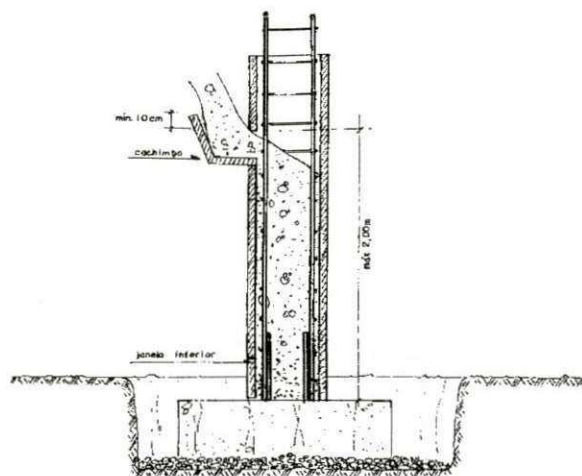
Figura 11. Concretagem de pilar
