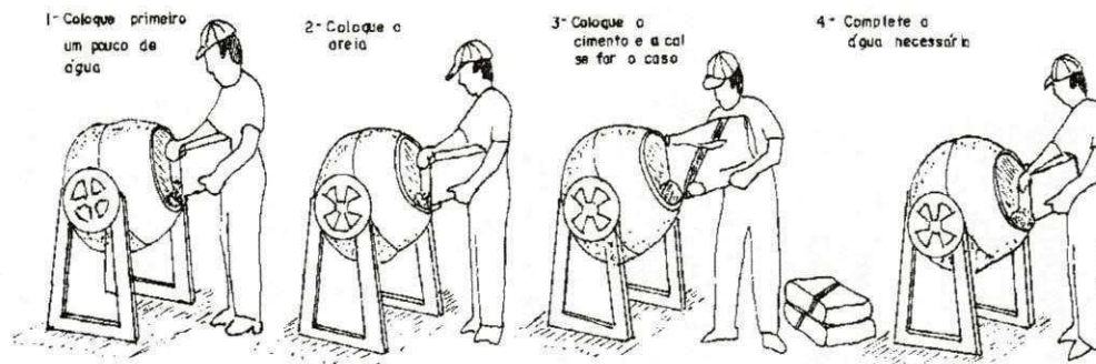
Figura 23. Preparação de argamassa com betoneira
