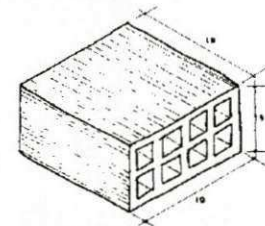
Figura 20. Tijolo furado
