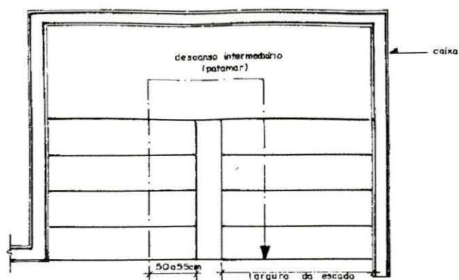
Figura 32. Indicação da escada
