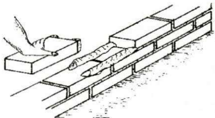
Figura 24. Aplicação de argamassa, tipo cordão
