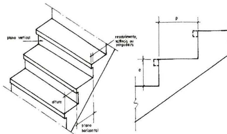
Figura 31. Detalhamento da escada
