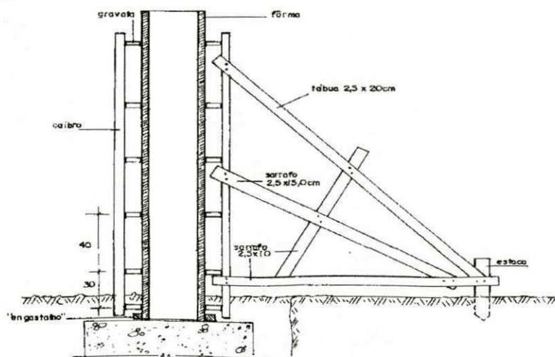
Figura 4. Escoramento de madeira para pilar
