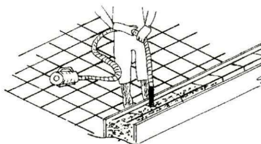
Figura 10. Demonstração do uso do vibrador
