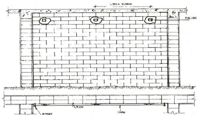
Figura 26. Assentamento de taliscas
