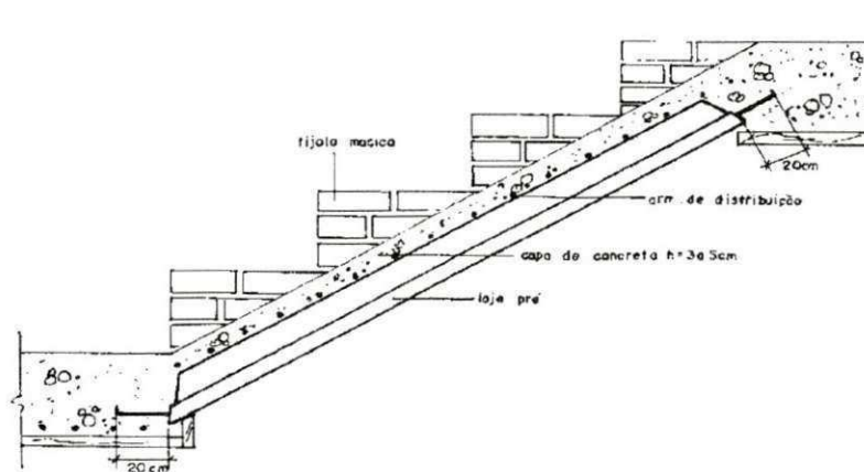
Figura 41. Concretagem da escada
