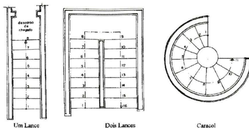
Figura 35. Modelos de escada
