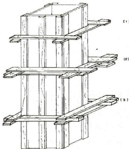
Figura 6. Tipos de gravatas mais usuais para pilares
