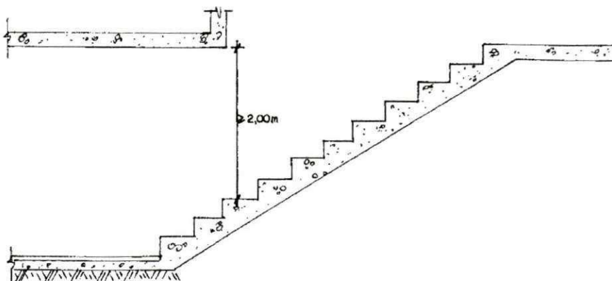
Figura 33. Altura mínima entre escadas
