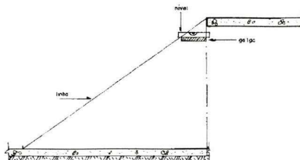
Figura 38. Marcação da escada
