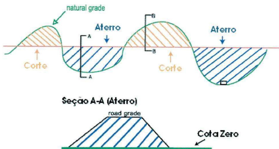
Figura 2: Esquema de aterro em terreno
