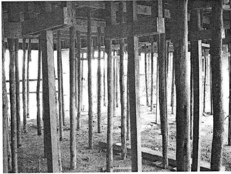
Figura 19 – Vista de baixo da fôrmas da laje na obra
