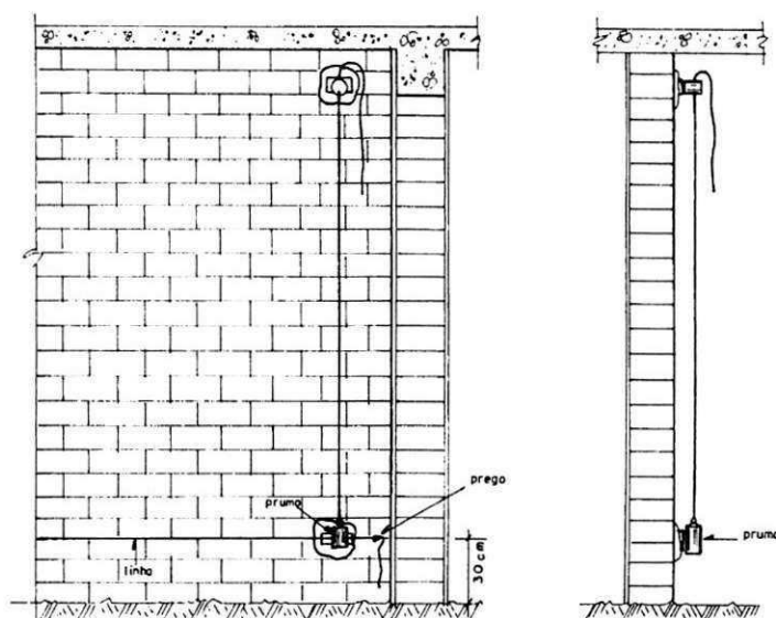
Figura 35 - Assentamento das taliscas inferiores
