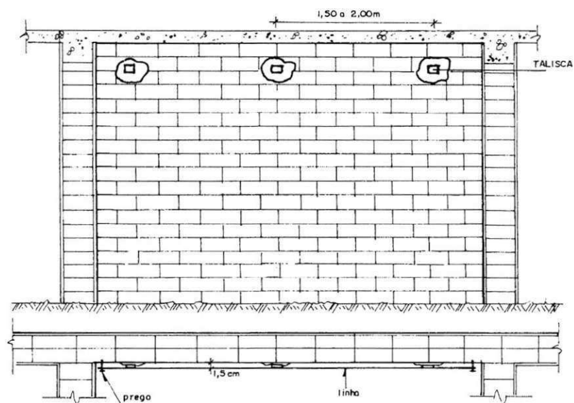
Figura 34 - Assentamento das taliscas superiores
