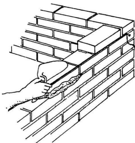
Figura 30 – Assentamento do tijolo
