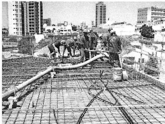
Figura 04 – Concretagem da laje com concreto usinado ou CDC
