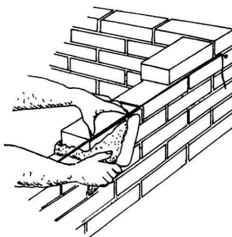
Figura 31 – Retirada do excesso de argamassa
