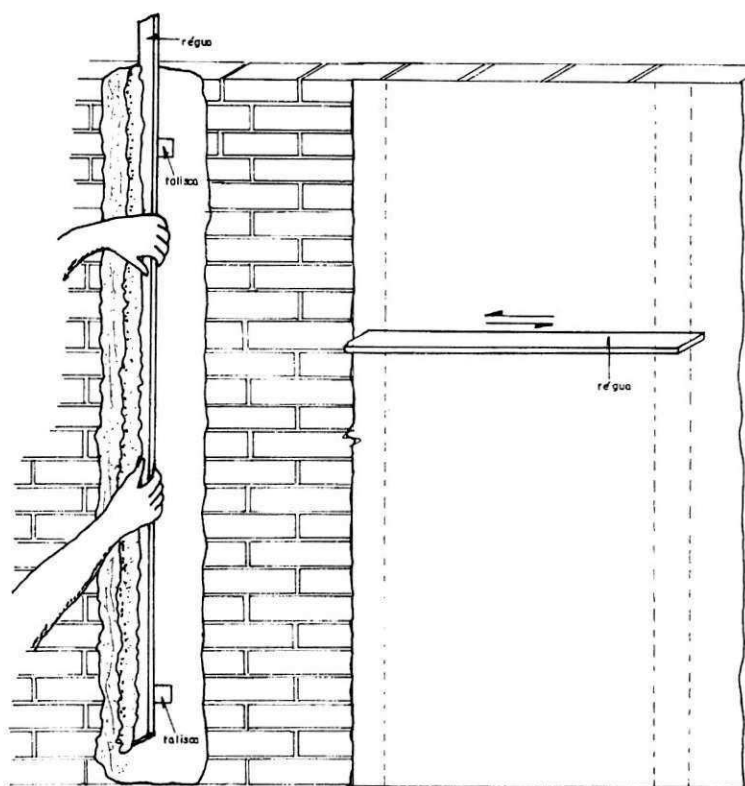
Figura 36 - Detalhe da execução das guias e do emboço
