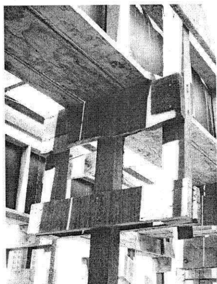
Figura 11 – Fôrmas das vigas
