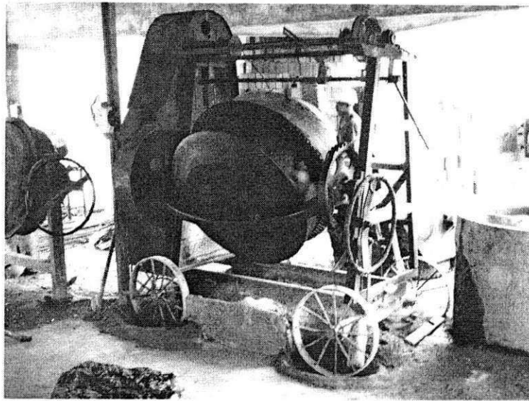
Figura 02 – Betoneira da obra
