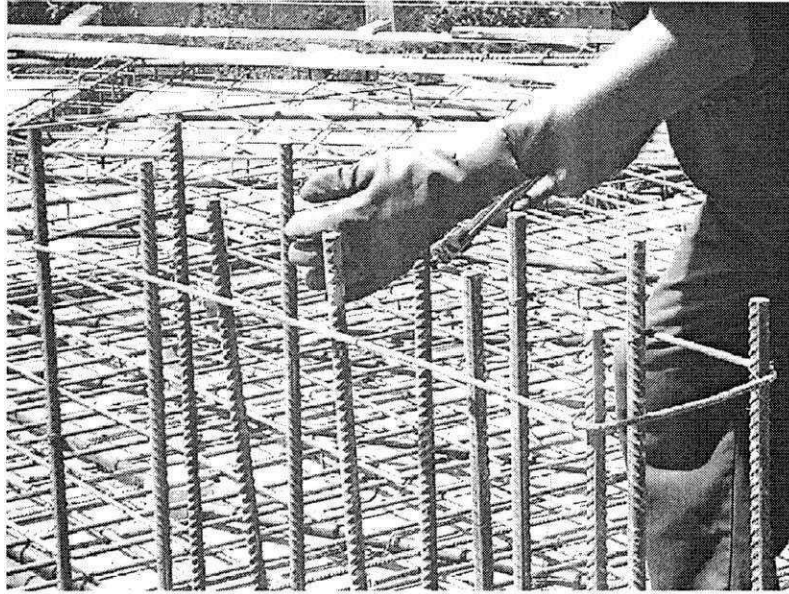
Figura 24 – Esqueleto do pilar
