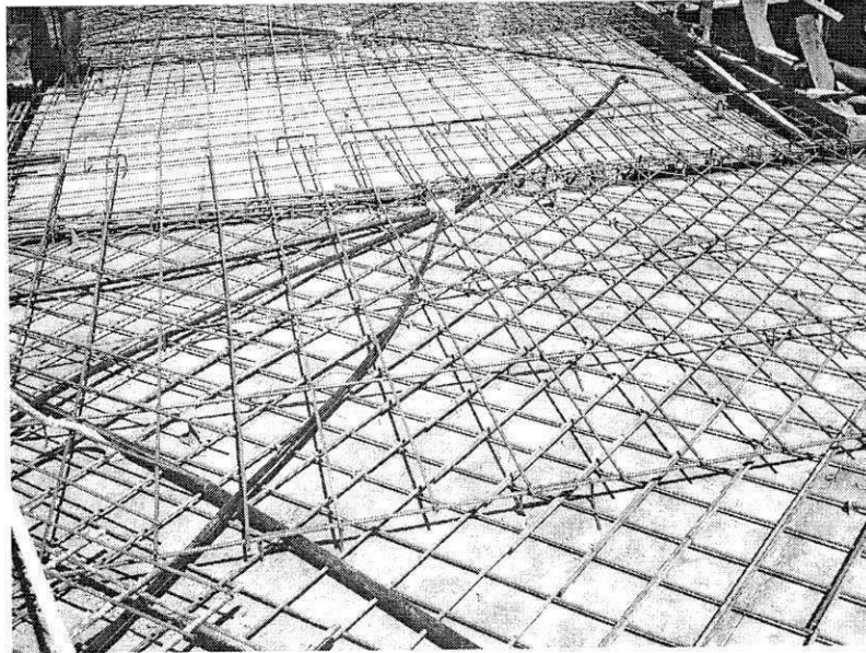
Figura 20 – Colocação das ferragens na laje da obra
