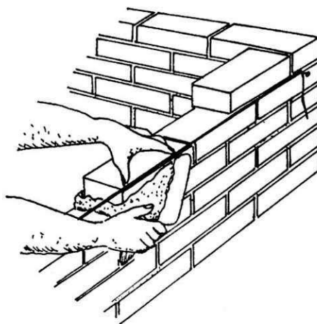
Figura 31 – Retirada do excesso de argamassa
