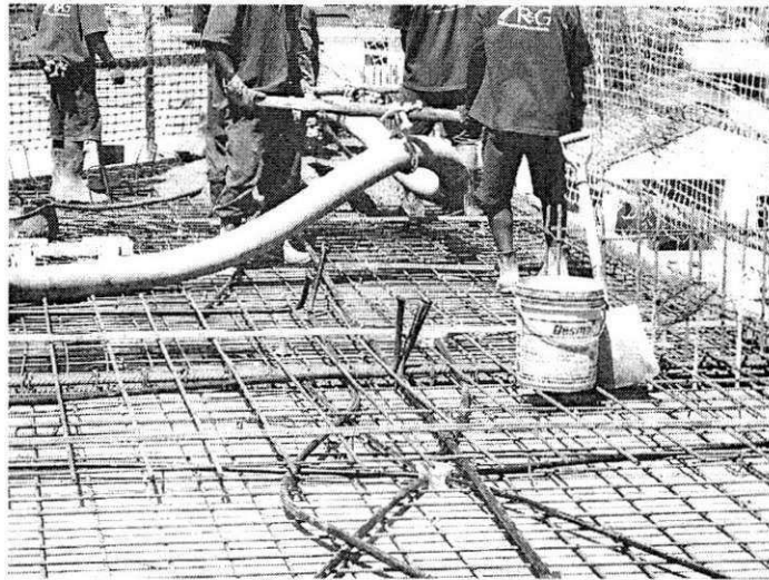
Figura 21 – Processo de concretagem da laje da obra
