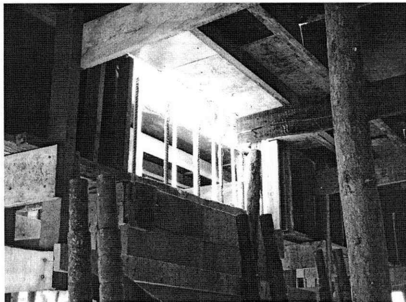
Figura 42 – Encontro do pilar com a viga
