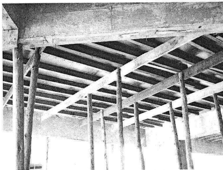
Figura 12 – Formas das Lajes
