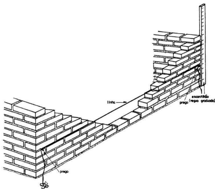
Figura 27 – Detalhe do nivelamento da elevação da alvenaria
