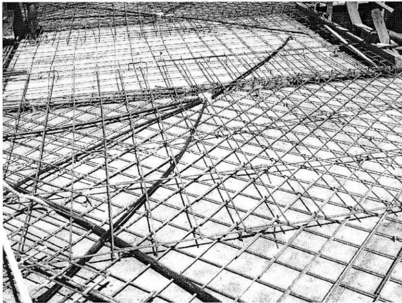
Figura 39 - Laje Maciça
