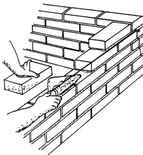
Figura 29 – Colocação da argamassa de assentamento
