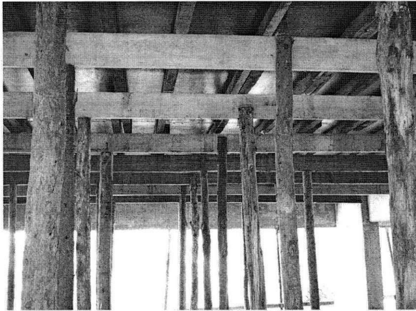
Figura 41 - Suporte de sustentação das fôrmas
