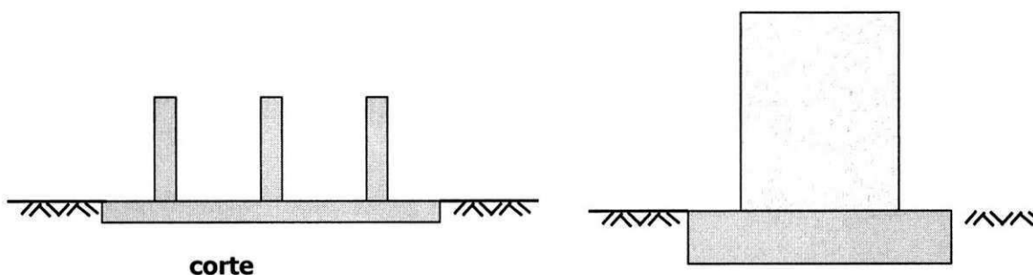
Figura 16 – Radier
