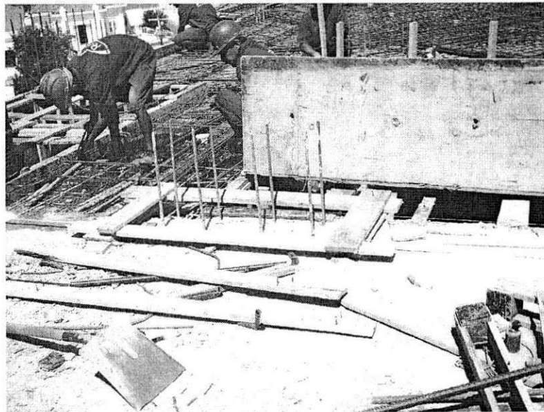
Figura 23 – Locação do pilares na Obra
