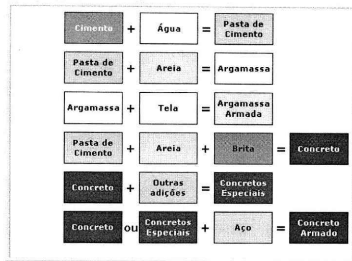
Figura 01 – Fluxograma de produção do concreto armado
