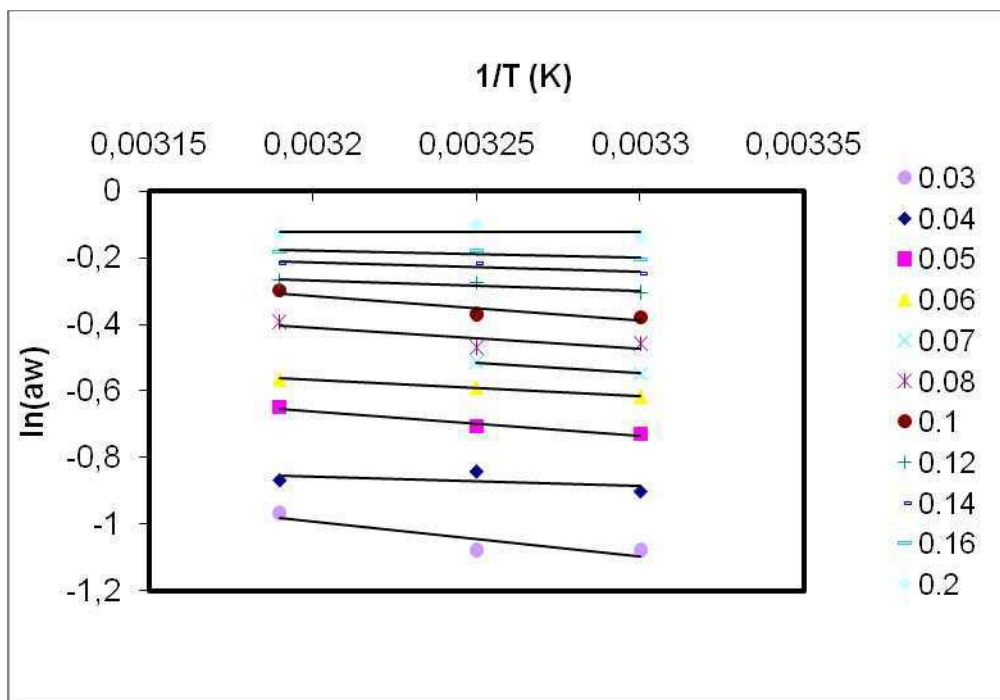
Figura 4.27. Curvas de \ln(a_w) versus 1/T , baseadas na equação de Clausius Clapeyron, para diferentes níveis de umidade.
