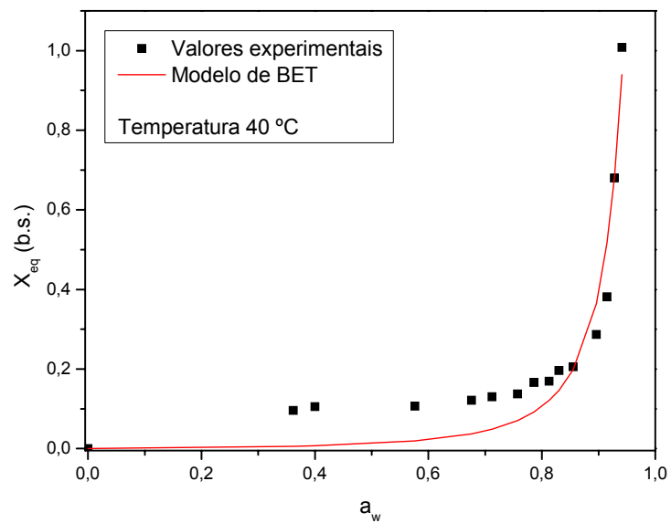
Figura 4.7. Isotherma de adsorção de umidade da palma forrageira in natura , na temperatura de 40 °C, ajustada pelo modelo de BET.
