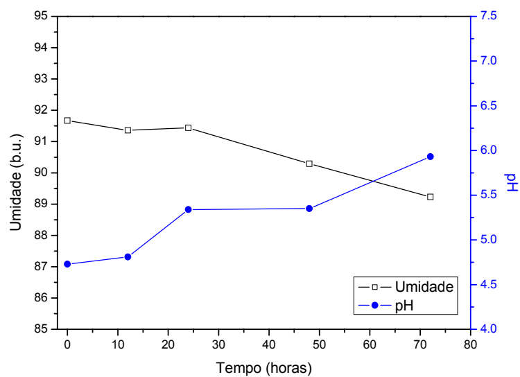
Figura 4A. Variação do pH e umidade em função do tempo de fermentação, a temperatura de 30 °C. Testes preliminares: experimento 4 (5% concentração inicial de leveduras).
