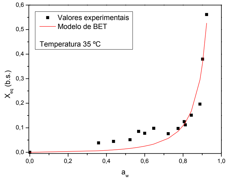
Figura 4.6. Isotherma de adsorção de umidade da palma forrageira in natura , na temperatura de 35 °C, ajustada pelo modelo de BET.
