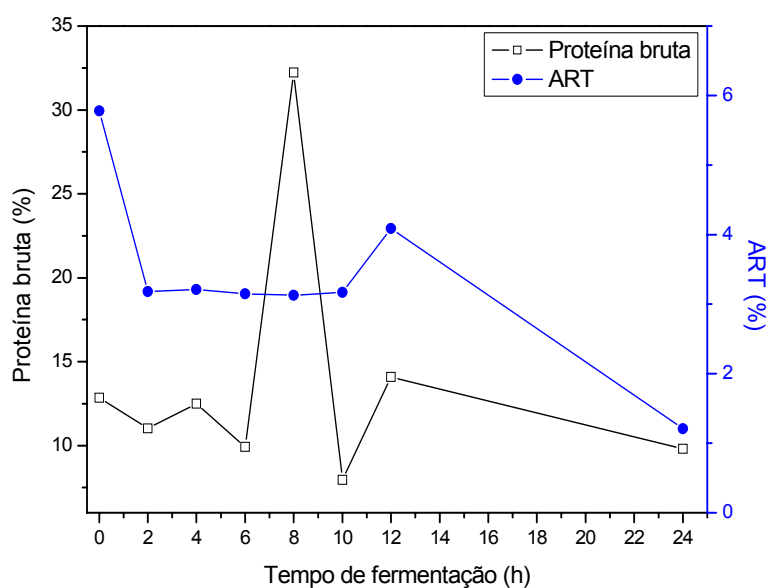
Figura 4.53. Perfil do percentual de proteína bruta e açúcares redutores totais durante a FSS da palma forrageira em tambor rotativo. Experimento 4.
