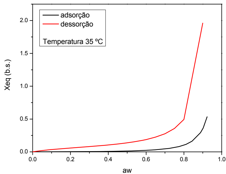
Figura 4.30. Histerese das isotermas de dessorção e adsorção de umidade da palma forrageira in natura , na temperatura 35 °C.
