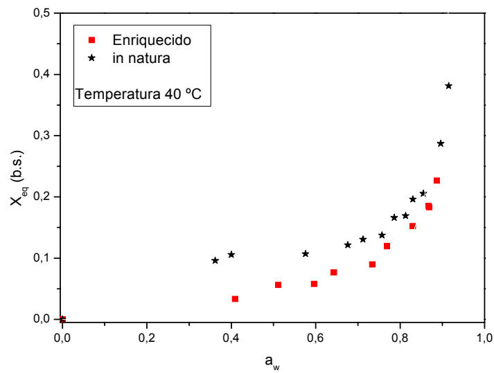
Figura 4.34. Isothermas de adsorção de umidade da palma forrageira in natura e enriquecida nutricionalmente, na temperatura de 40 °C.
