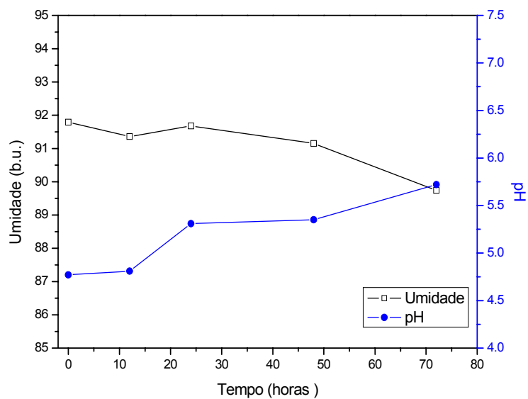
Figura 3A. Variação do pH e umidade em função do tempo de fermentação, a temperatura de 30 °C. Testes preliminares: experimento 3 (1% concentração inicial de leveduras).
