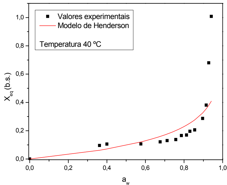
Figura 4.10. Isoterma de adsorção de umidade da palma forrageira in natura , na temperatura de 40 °C, ajustada pelo modelo de Henderson.
