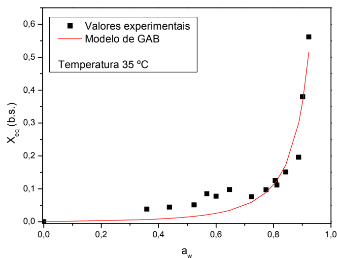
Figura 4.3. Isoterma de adsorção de umidade da palma forrageira in natura , na temperatura de 35 °C, ajustada pelo modelo de GAB.
