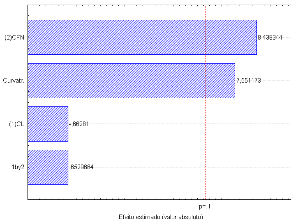
Figura 4.60. Gráfico de Pareto para o percentual de proteína bruta, após 4 h de fermentação em biorreator tambor rotativo.
