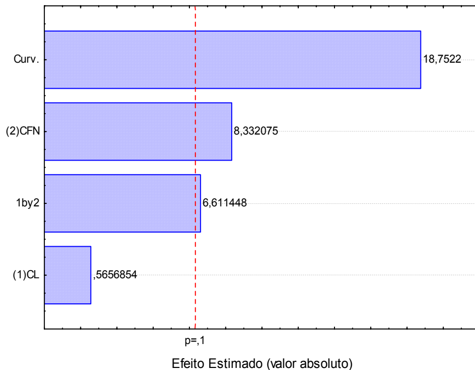
Figura 4.56. Gráfico de Pareto para o percentual de proteína bruta, após 8 h de fermentação em biorreator bandeja.
