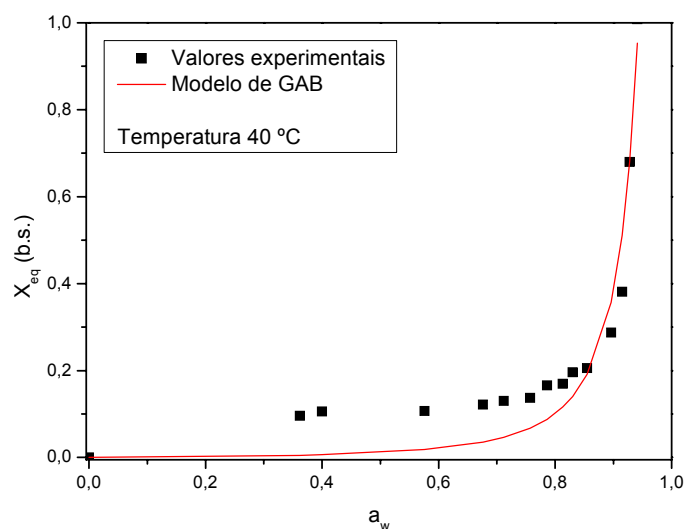
Figura 4.4. Isoterma de adsorção de umidade da palma forrageira in natura , na temperatura de 40 °C, ajustada pelo modelo de GAB.
