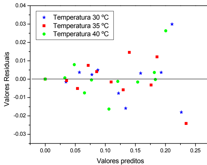
Figura 4.26. Distribuição dos resíduos para o modelo de Henderson, em função dos valores preditos.
