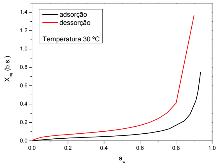
Figura 4.29. Histerese das isotermas de dessorção e adsorção de umidade da palma forrageira in natura , na temperatura 30 °C.
