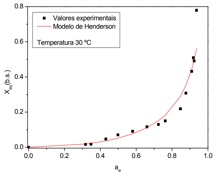
Figura 4.8. Isoterma de adsorção de umidade da palma forrageira in natura , na temperatura de 30 °C, ajustada pelo modelo de Henderson.
