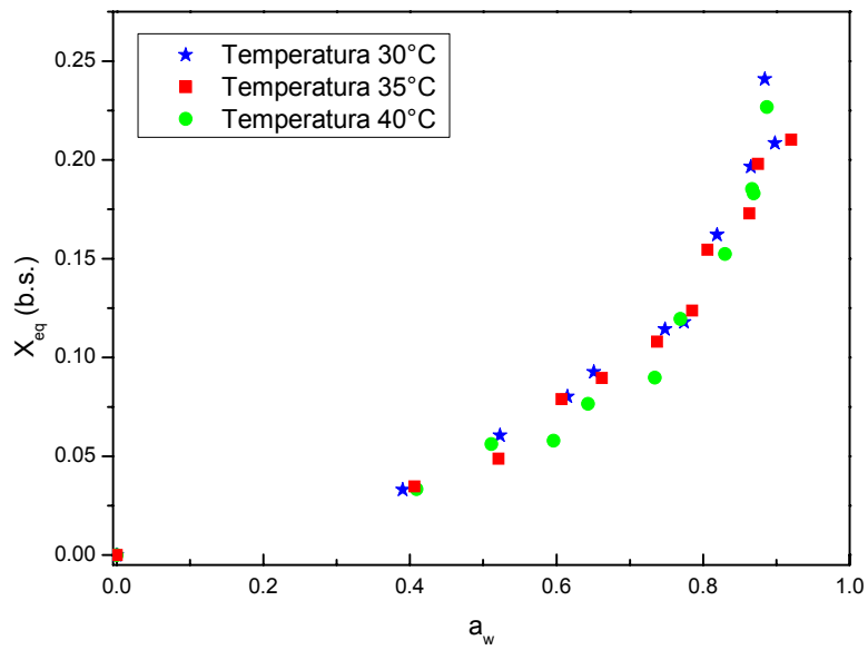
Figura 4.14. Influência da temperatura nas isotermas de adsorção de umidade da palma forrageira enriquecida nutricionalmente.
