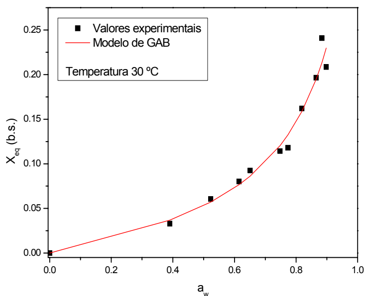
Figura 4.15. Isoterma de adsorção de umidade da palma forrageira enriquecida nutricionalmente, na temperatura de 30 °C, ajustada pelo modelo de GAB.
