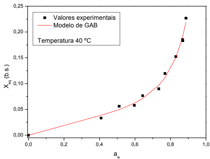
Figura 4.17. Isotherma de adsorção de umidade da palma forrageira enriquecida nutricionalmente, na temperatura de 40 °C, ajustada pelo modelo de GAB.
