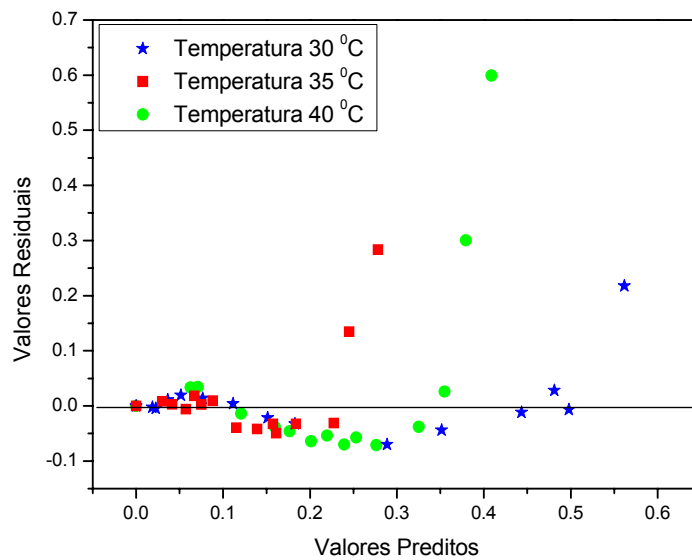
Figura 4.13. Distribuição dos resíduos para o modelo de Henderson, em função dos valores preditos.
