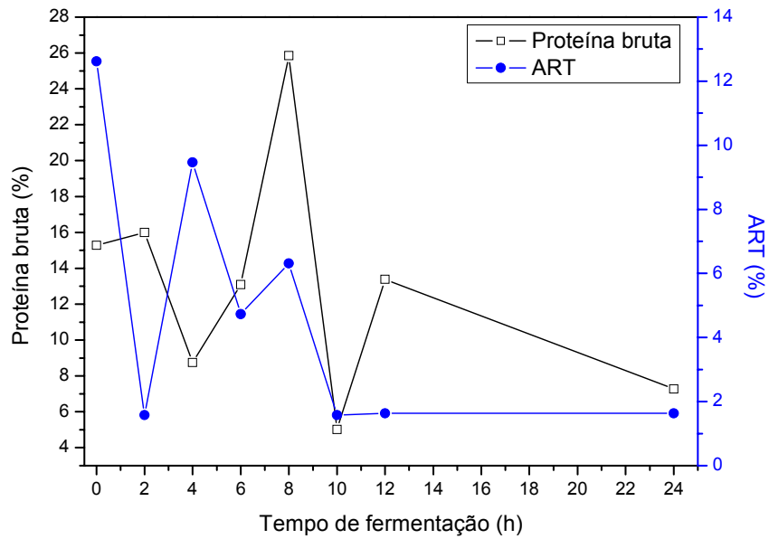
Figura 4.47. Perfil do percentual de proteína bruta e açúcares redutores totais durante a FSS da palma forrageira em bandeja. Experimento 4.
