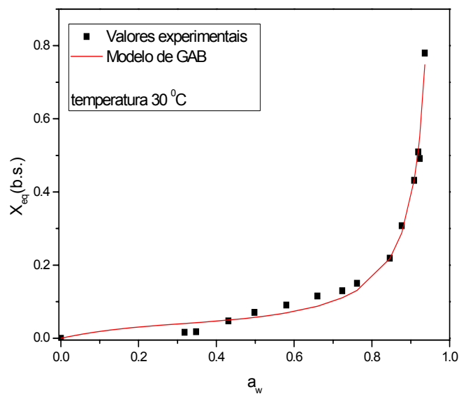
Figura 4.2. Isotherma de adsorção de umidade da palma forrageira in natura , na temperatura de 30 °C, ajustada pelo modelo de GAB.
