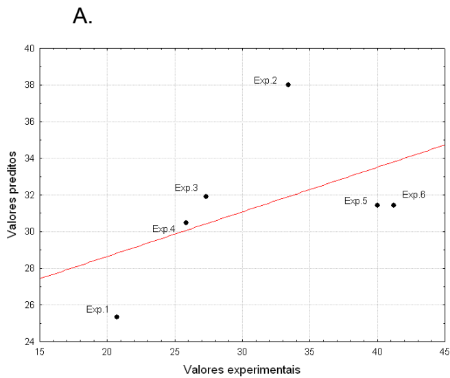
Figura 4.58. Valores de proteína bruta observados experimentalmente versus valores preditos pelo modelo matemático linear sem curvatura (A) e com curvatura (B), no tempo de 8 h.
