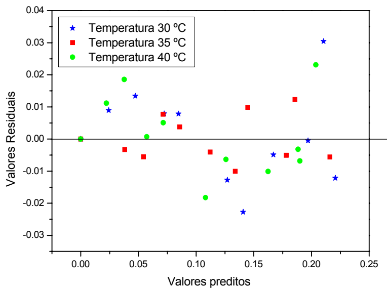
Figura 4.25. Distribuição dos resíduos para o modelo de BET, em função dos valores preditos.
