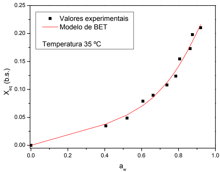
Figura 4.19. Isotherma de adsorção de umidade da palma forrageira enriquecida nutricionalmente, na temperatura de 35 °C, ajustada pelo modelo de BET.
