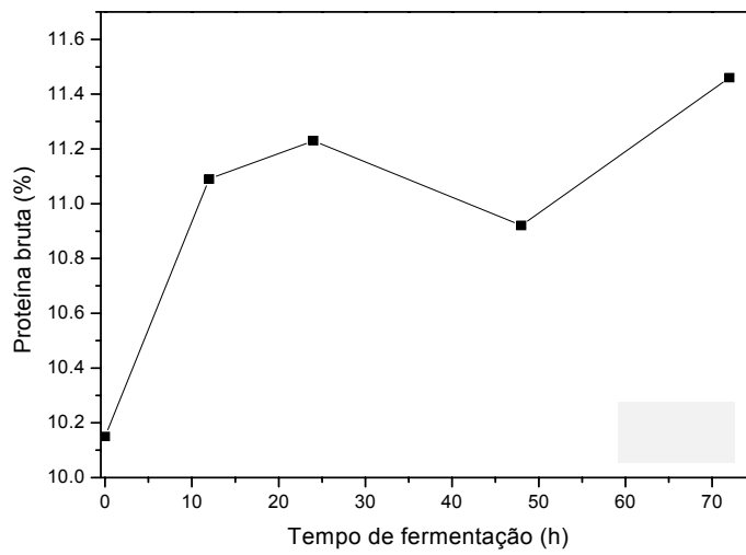
Figura 4.37. Perfil do percentual de proteína bruta durante a FSS da palma forrageira, testes preliminares, Experimento 3.
