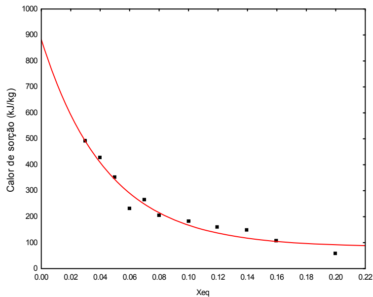
Figura 4.28. Calor isostérico de adsorção em função da umidade da palma forrageira enriquecida nutricionalmente (os pontos representam os dados experimentais e a linha o modelo estudado).
