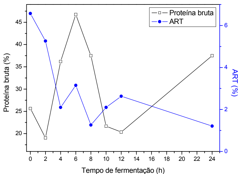
Figura 4.51. Perfil do percentual de proteína bruta e açúcares redutores totais durante a FSS da palma forrageira em tambor rotativo. Experimento 2.
