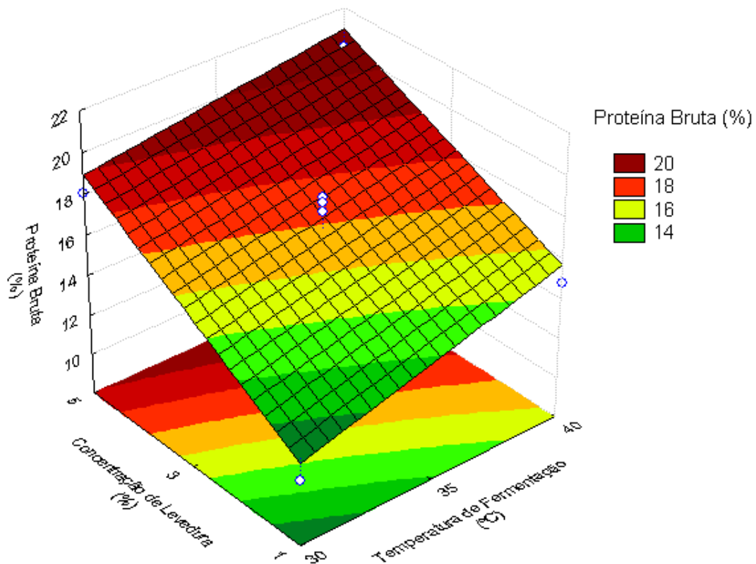
Figura 4.42. Influência das variáveis independentes, temperatura de fermentação e concentração inicial de leveduras, sobre o teor de proteína bruta da palma forrageira.
