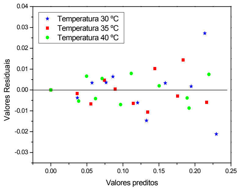
Figura 4.24. Distribuição dos resíduos para o modelo de GAB, em função dos valores preditos.
