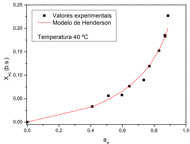
Figura 4.23. Isotherma de adsorção de umidade da palma forrageira enriquecida nutricionalmente, na temperatura de 40 °C, ajustada pelo modelo de Henderson.
