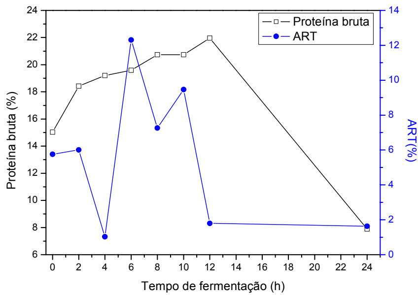
Figura 4.44. Perfil do percentual de proteína bruta e açúcares redutores totais durante a FSS da palma forrageira em bandeja. Experimento 1.
