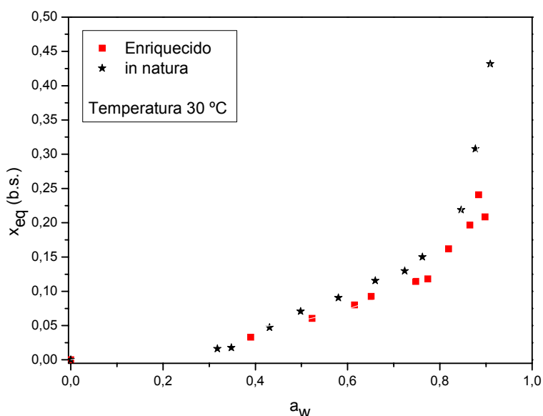
Figura 4.32. Isotermas de adsorção de umidade da palma forrageira in natura e enriquecida nutricionalmente, na temperatura de 30 °C.
