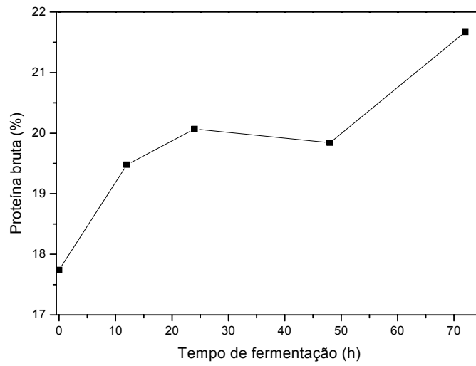
Figura 4.36. Perfil do percentual de proteína bruta durante a FSS da palma forrageira, testes preliminares, Experimento 2.
