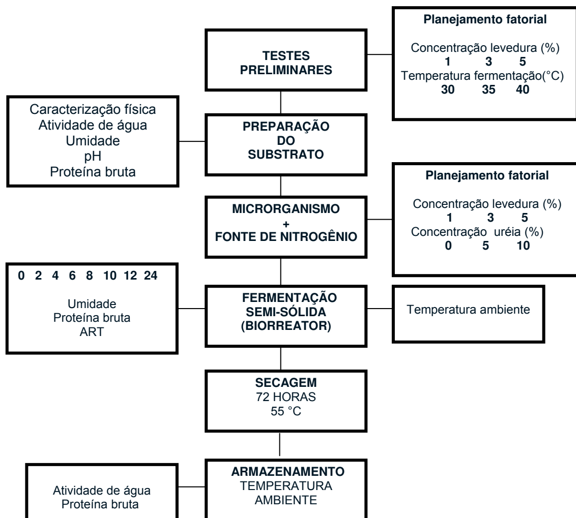
Figura 3.1. Etapas do processo de enriquecimento nutricional da palma forrageira.
