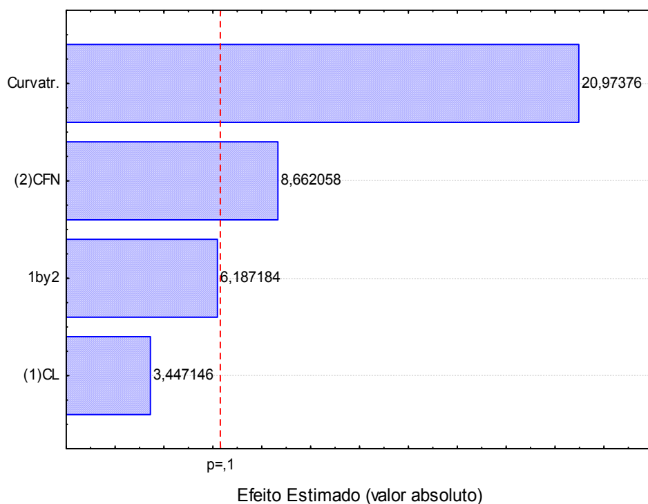
Figura 4.57. Gráfico de Pareto para o aumento protéico, após 8 h de fermentação em biorreator bandeja.
