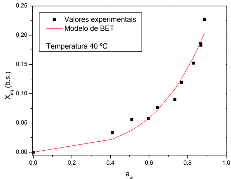
Figura 4.20. Isotherma de adsorção de umidade da palma forrageira enriquecida nutricionalmente, na temperatura de 40 °C, ajustada pelo modelo de BET.
