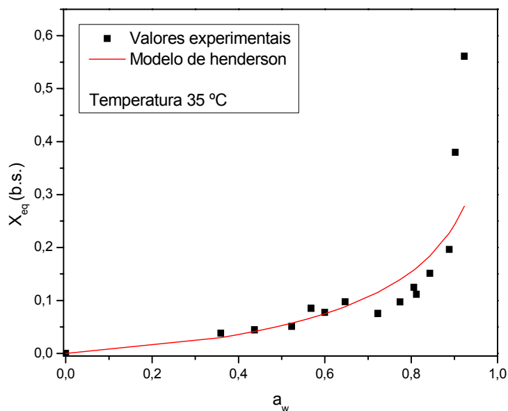
Figura 4.9. Isoterma de adsorção de umidade da palma forrageira in natura , na temperatura de 35 °C, ajustada pelo modelo de Henderson.
