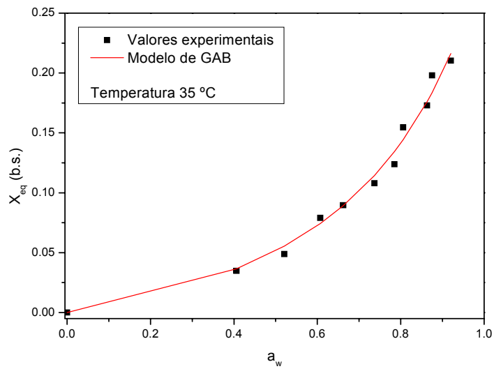
Figura 4.16. Isotherma de adsorção de umidade da palma forrageira enriquecida nutricionalmente, na temperatura de 35°C, ajustada pelo modelo de GAB.
