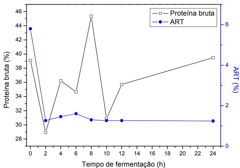
Figura 4.52. Perfil do percentual de proteína bruta e açúcares redutores totais durante a FSS da palma forrageira em tambor rotativo. Experimento 3.
