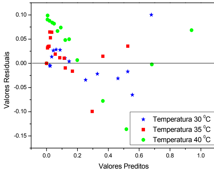
Figura 4.12. Distribuição dos resíduos para o modelo de BET, em função dos valores preditos.
