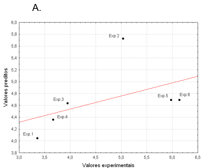
Figura 4.59. Valores de aumentos protéicos observados experimentalmente versus valores preditos pelo modelo matemático linear sem curvatura (A) e com curvatura (B), no tempo de 8 h.
