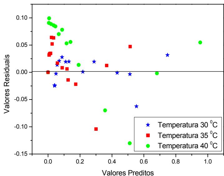
Figura 4.11. Distribuição dos resíduos para o modelo de GAB, em função dos valores preditos.
