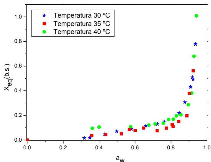
Figura 4.1. Influência da temperatura nas isotermas de adsorção de umidade da palma forrageira in natura .
