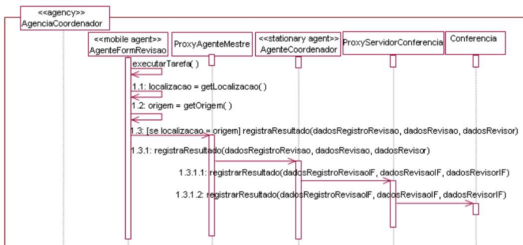
Figura 7.6: Diagrama de seqüência dependente de plataforma da operação aprovarRevisao – Parte 2
