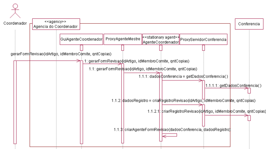
Figura 7.1: Diagrama de sequência dependente de plataforma da operação gerarFormRevisao – Parte 1
