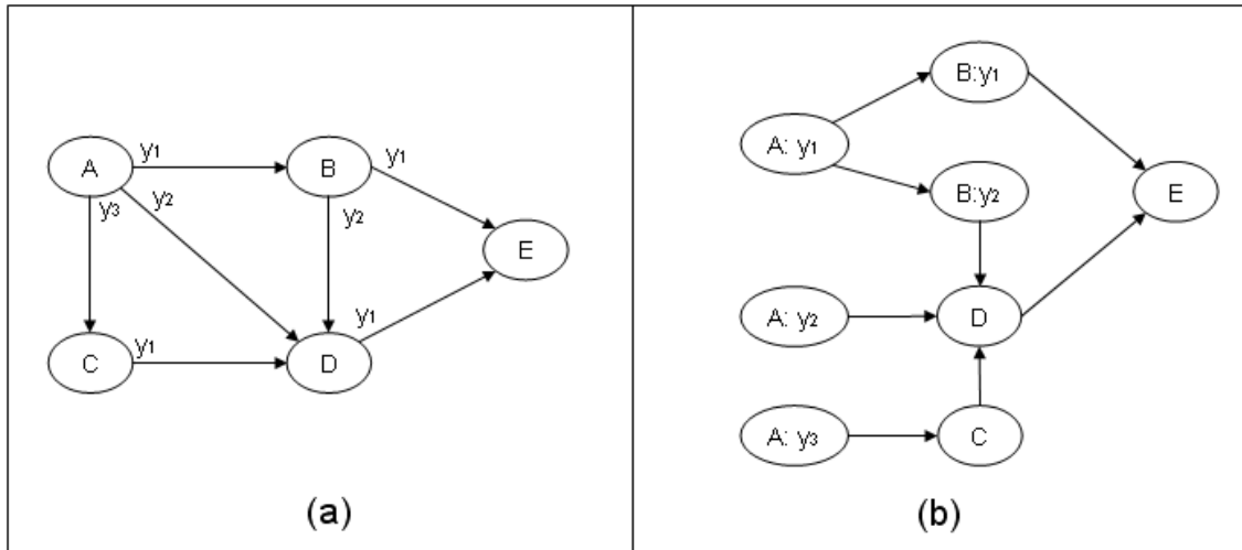
Figura 12: Modelo de propagação de falhas para um sistema com componentes de múltipla saídas
