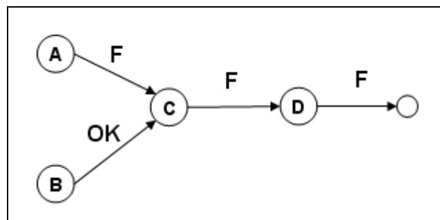
Figura 14: Exemplo de um FPM para um determinado sistema
