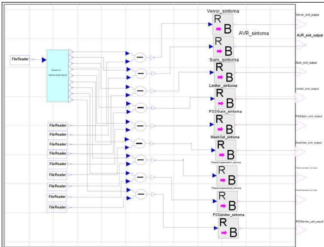
Figura 45: Modelo de Detecção para o sistema de excitação
