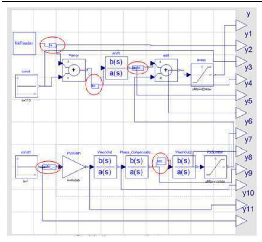
Figura 96: Modelo do Sistema de Excitação com componentes de injeção de falha
