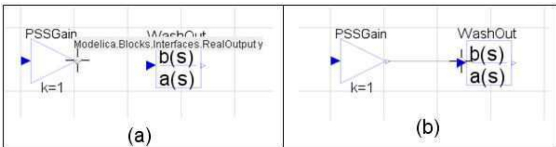
Figura 58: Conectando componentes no SimForge.
