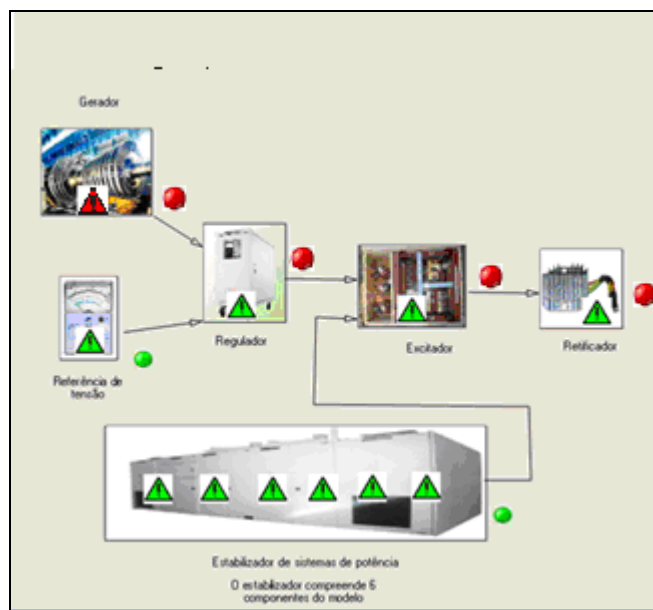
Figura 34: Auto-FDI Editor – Diferença entre os componentes de alarme
