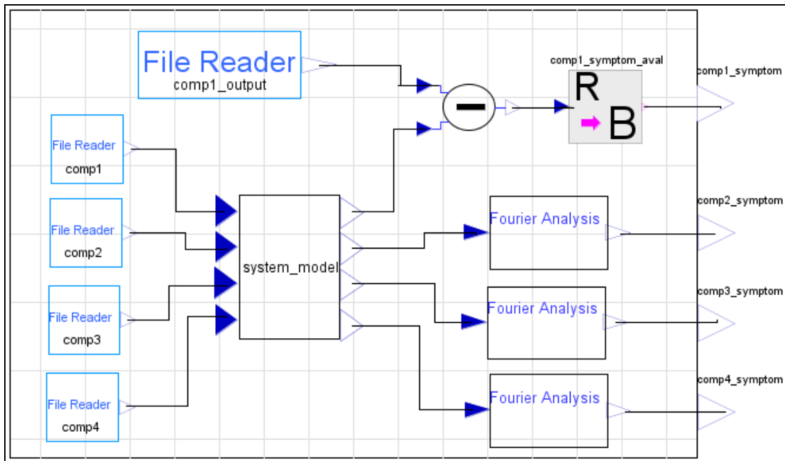
Figura 47: Detecção de falhas usando técnicas baseadas em modelo do sistema e modelo de sinais
