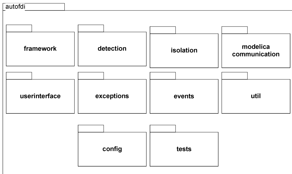
Figura 40: Principais pacotes da ferramenta Auto-FDI
