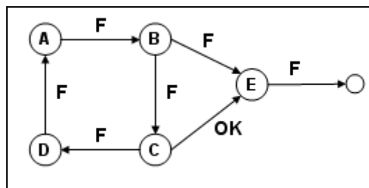
Figura 16: Exemplo de FPM com propagação de falhas em um ciclo
