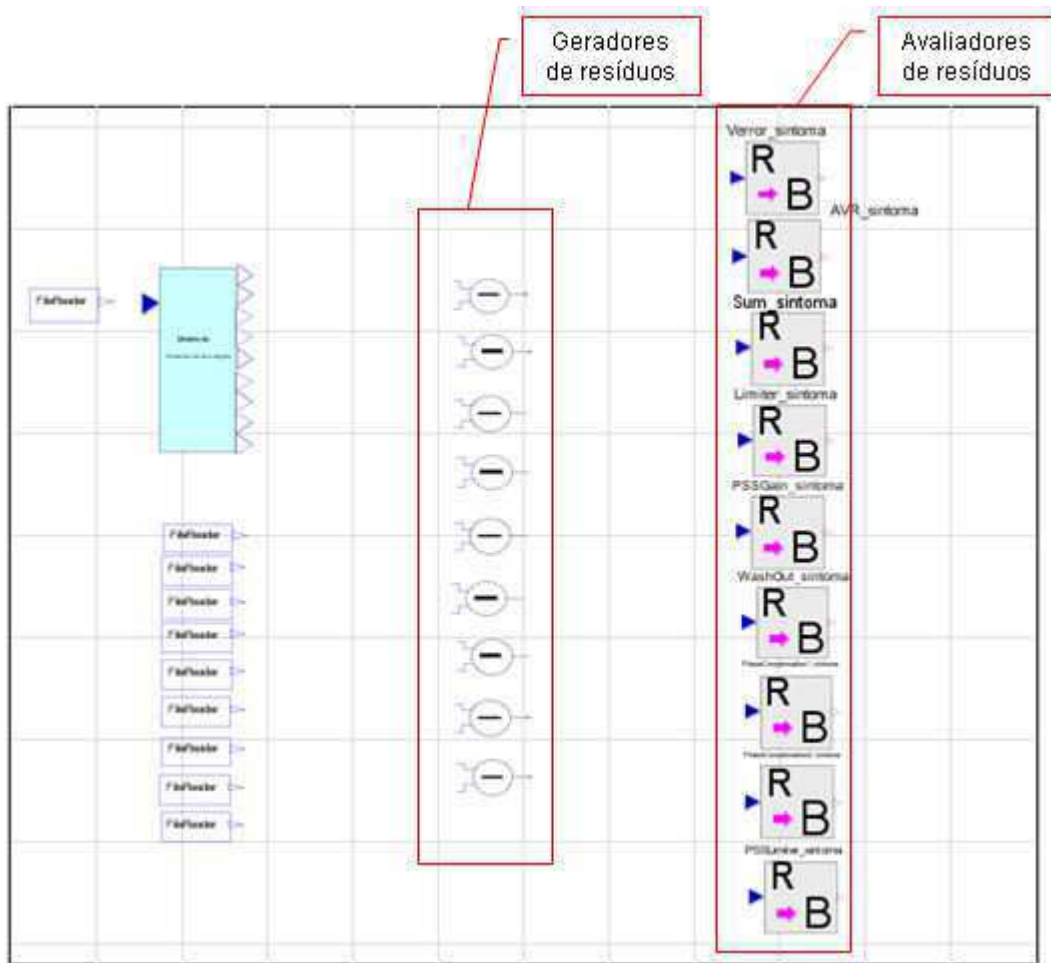
Figura 74: Modelo de detecção de falhas – adição dos geradores e dos adaptadores de resíduos
