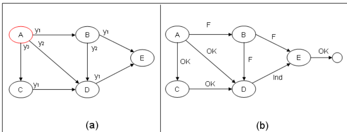
Figura 13: Modelo de propagação de falha para um determinado sistema
