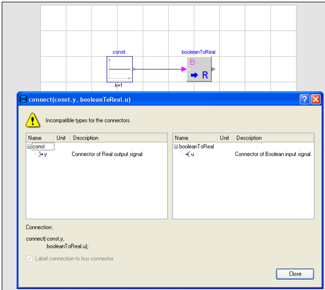
Figura 44: Verificação de inconsistências no modelo
