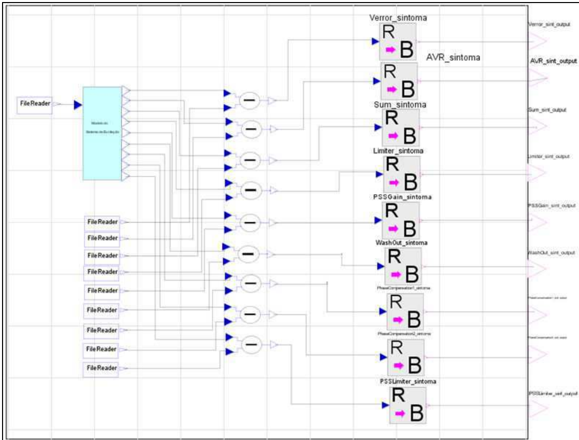
Figura 75: Modelo de detecção de falhas finalizado
