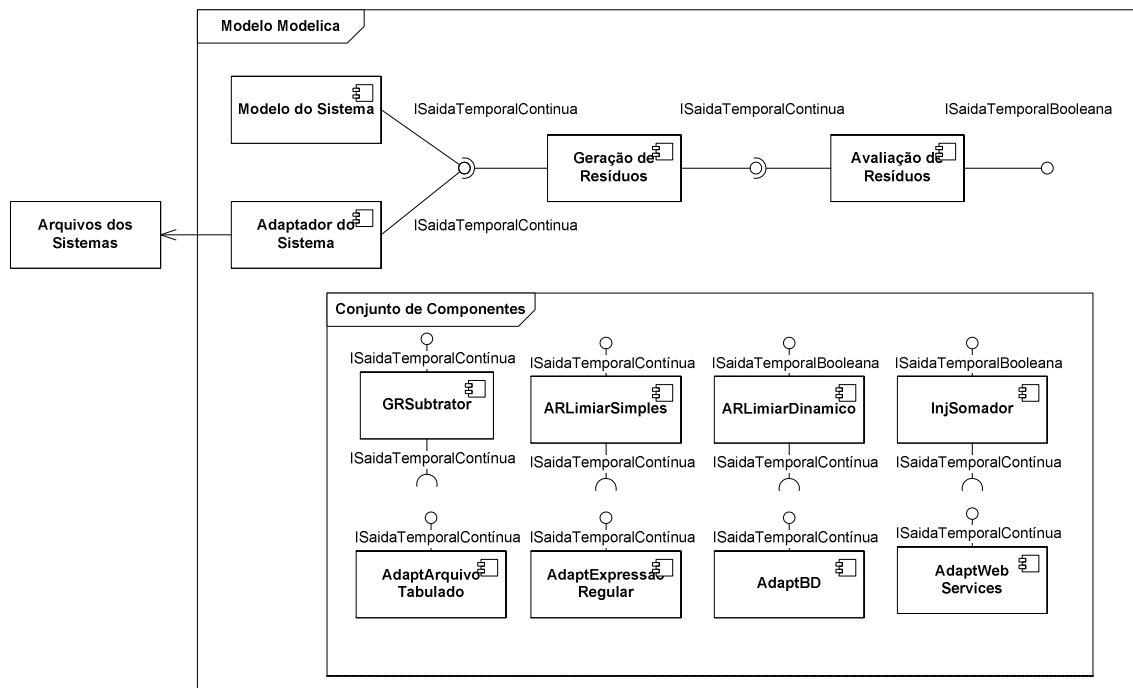
Figura 26: Arquitetura: Modelo de Detecção
