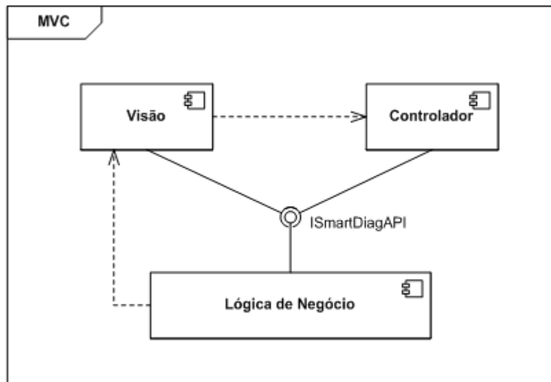
Figura 24: Padrão Model-View-Controller
