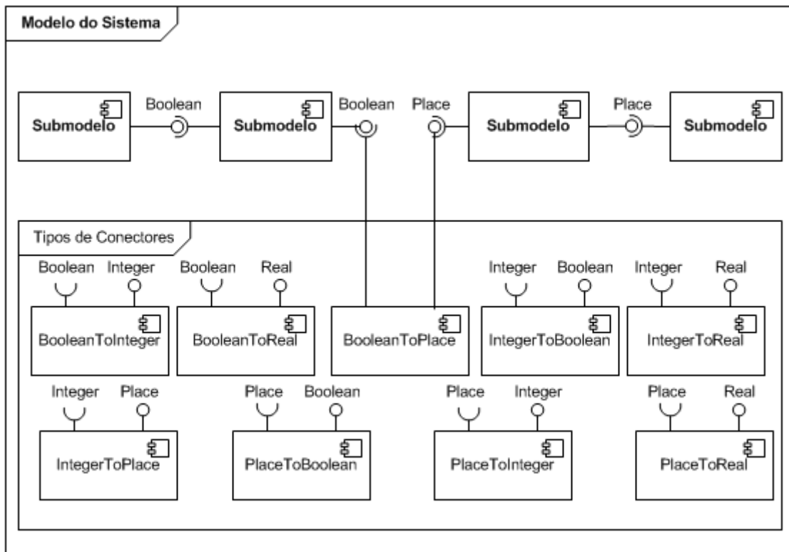
Figura 27: Arquitetura: Modelo do Sistema
