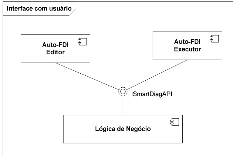
Figura 23: Arquitetura: Interface com o usuário
