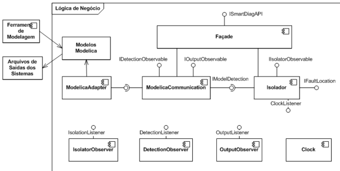
Figura 25: Arquitetura: Lógica de negócio
