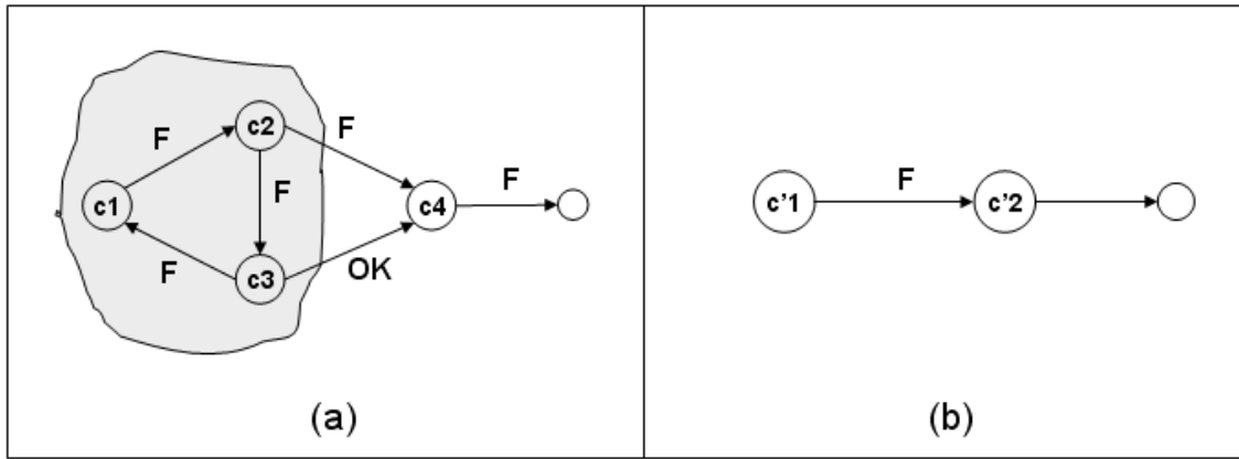
Figura 19: Redução do grafo (Exemplo 1)
