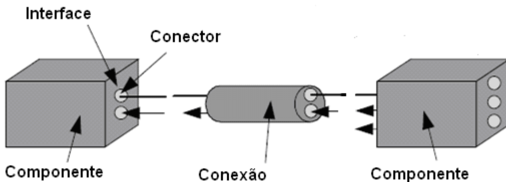
Figura 29: Mecanismo de conexão da linguagem Modelica
