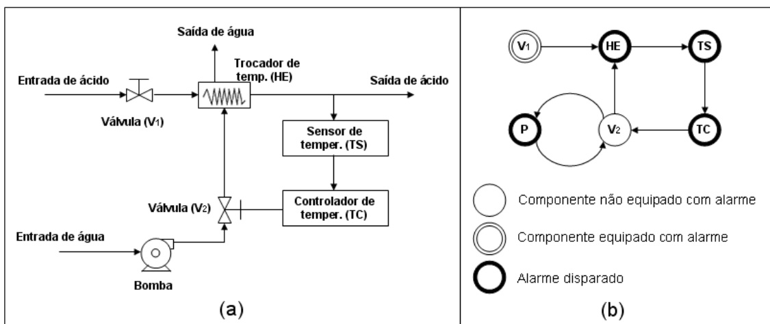
Figura 11 (retirada de [Rao1993]): Sistema de esfriamento de ácido nítrico. (a) Diagrama de bloco funcional. (b). Modelo de propagação de falhas.
