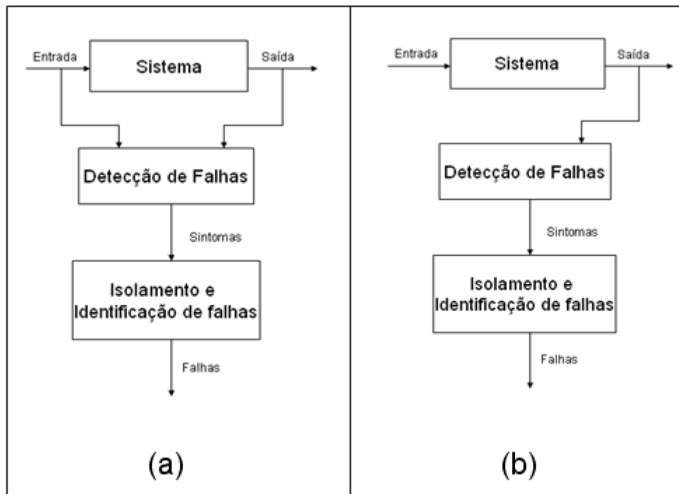
Figura 4 (retirada de [Pontes2008]): Estrutura de um sistema de detecção e diagnóstico de falhas baseado em modelos
