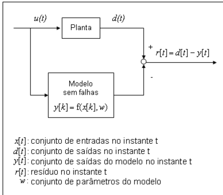
Figura 6 (baseada em [Munoz1996]): Geração de resíduos baseada no modelo de funcionamento normal da planta do sistema
