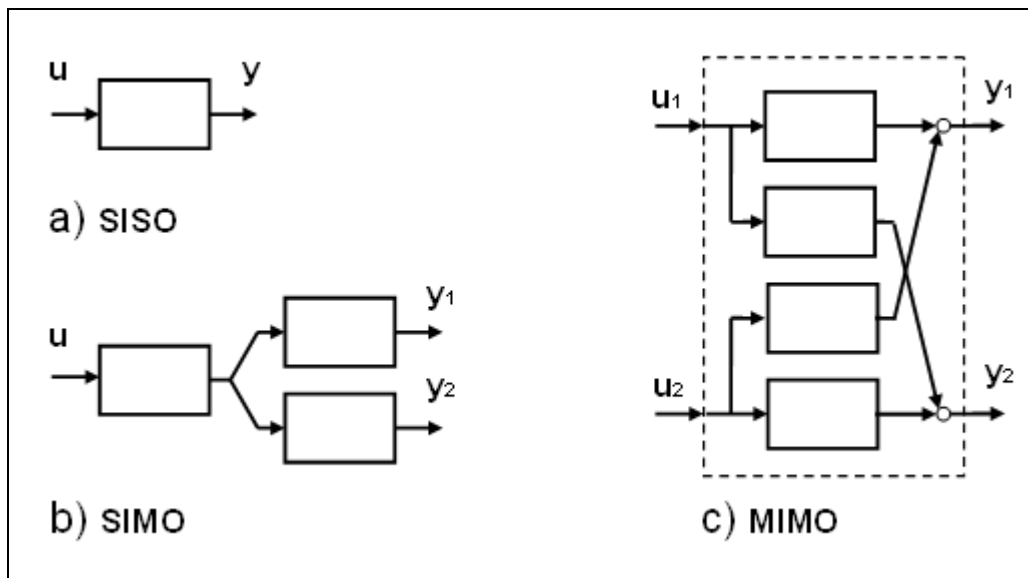
Figura 10: Classificação de sistemas de acordo com a quantidade de entradas e saídas
