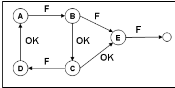
Figura 17: Exemplo de FPM sem propagação de falhas no ciclo
