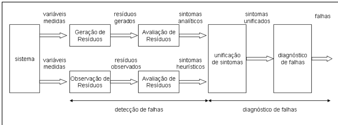
Figura 7 (baseada em [Isermann2006]): Unificação de sintomas no processo de detecção e diagnóstico de falhas
