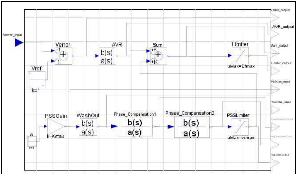
Figura 54: Representação visual do modelo do sistema de excitação do tipo ST1A
