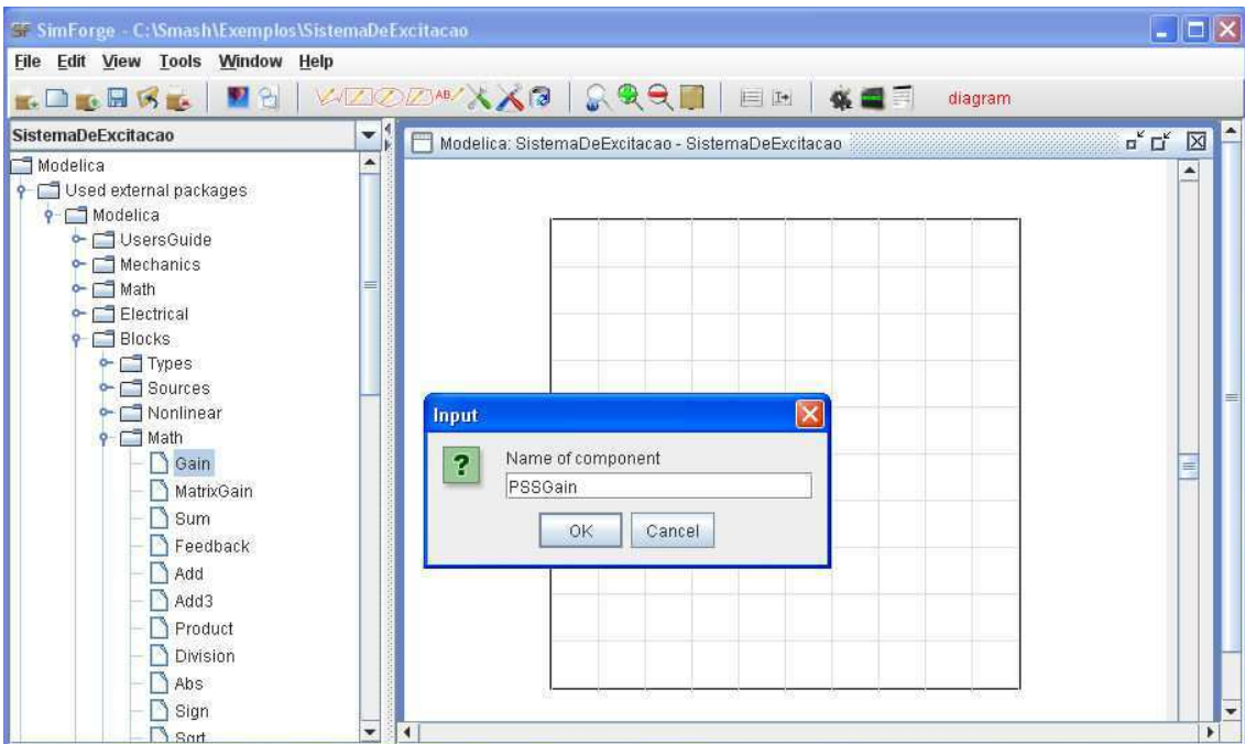
Figura 55: Inserindo o componente PSSGain
