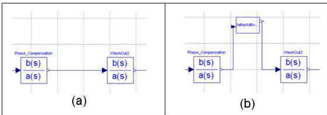
Figura 97: Injeção de Falhas: (a) modelo sem componente de injeção de falha; (b) modelo com componente de injeção de falha
