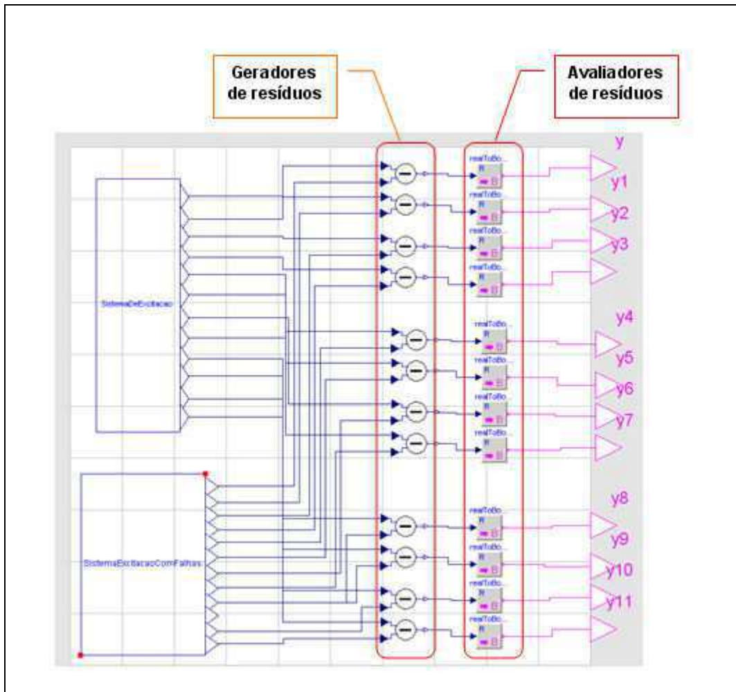
Figura 95: Modelo de Detecção para o Sistema de Excitação
