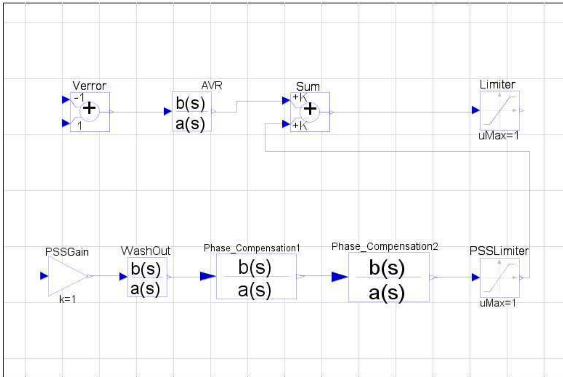
Figura 59: Modelo parcial do sistema de excitação
