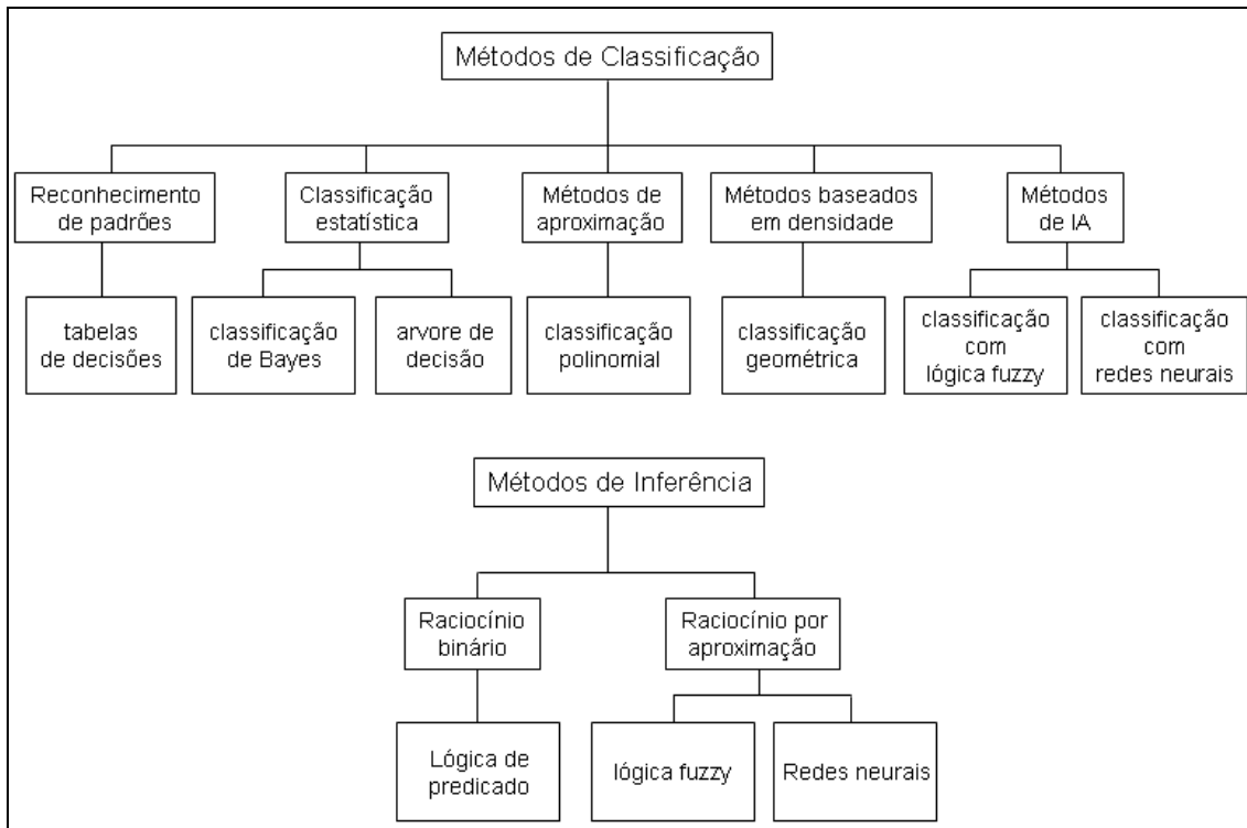
Figura 8: Métodos de isolamento e identificação de falhas
