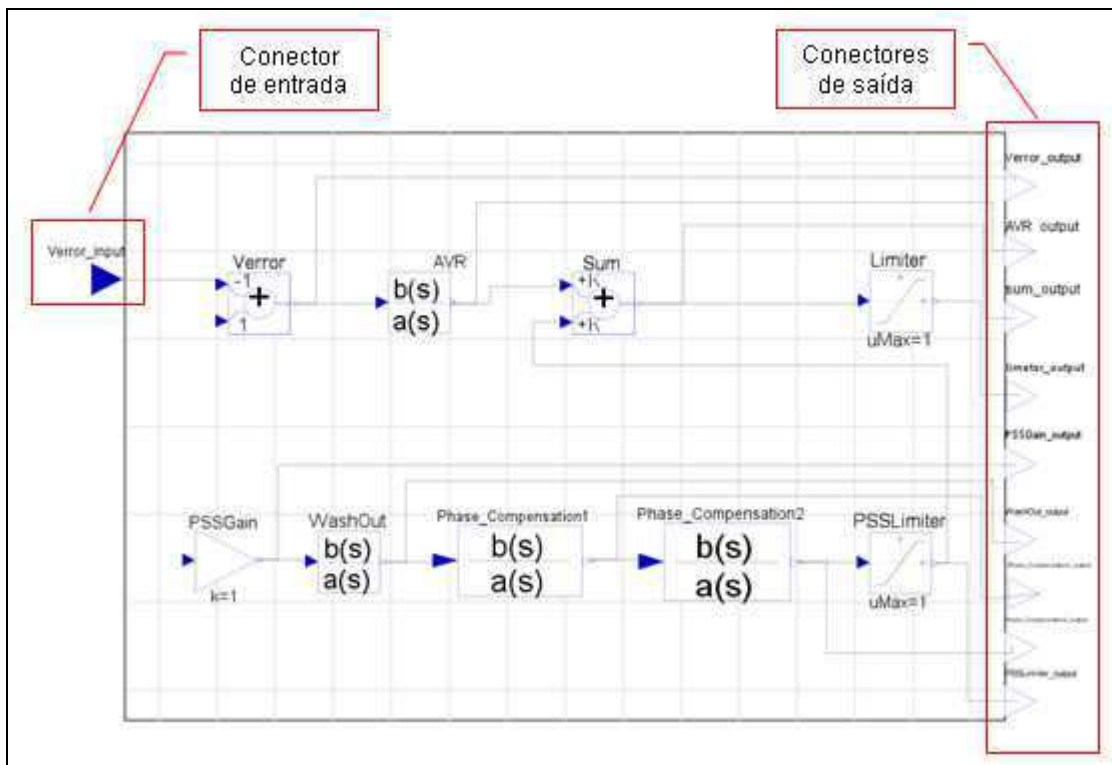
Figura 62: Modelo parcial do sistema de excitação
