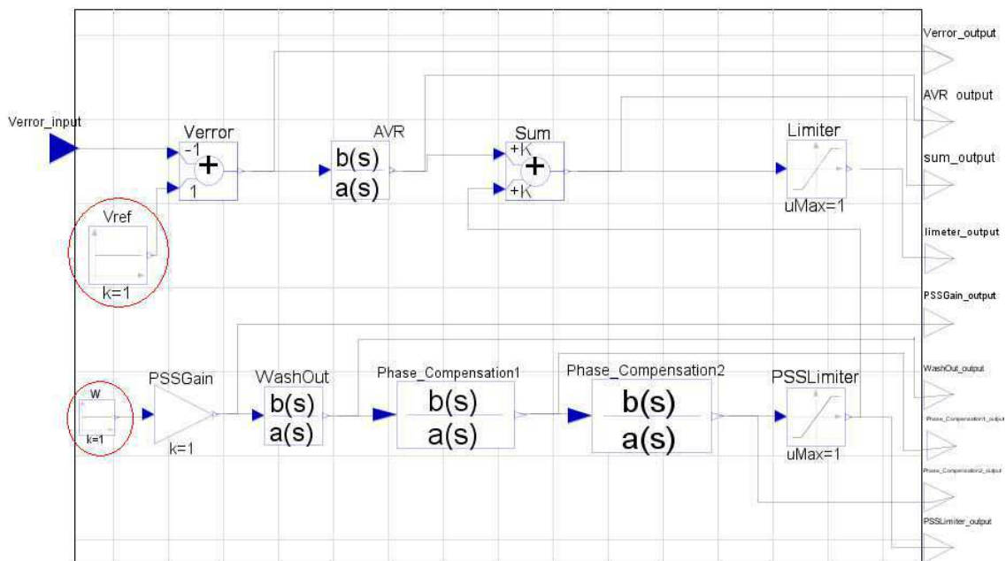
Figura 64: Modelo parcial do sistema de excitação
