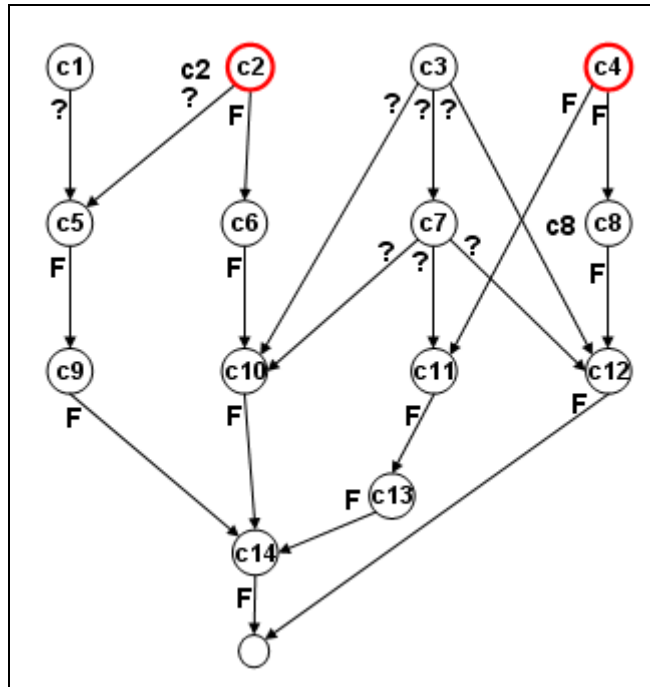
Figura 18 (retirada de [CS2001]): FPM para um determinado sistema
