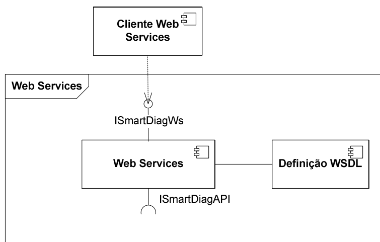
Figura 28: Arquitetura: Web Services
