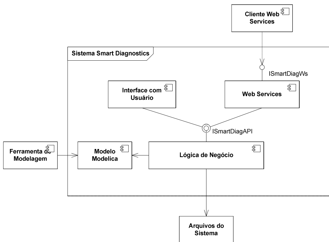
Figura 22: Arquitetura geral do Auto-FDI
