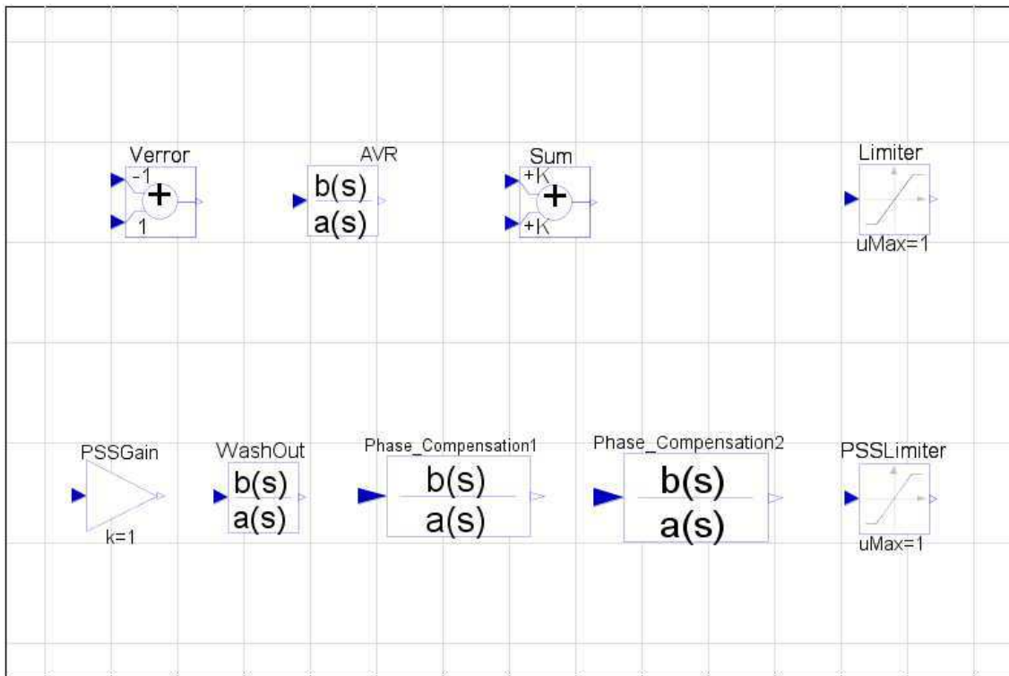
Figura 57: Modelo parcial do sistema de excitação.
