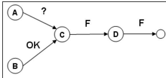
Figura 15: Exemplo de um FPM para um determinado sistema
