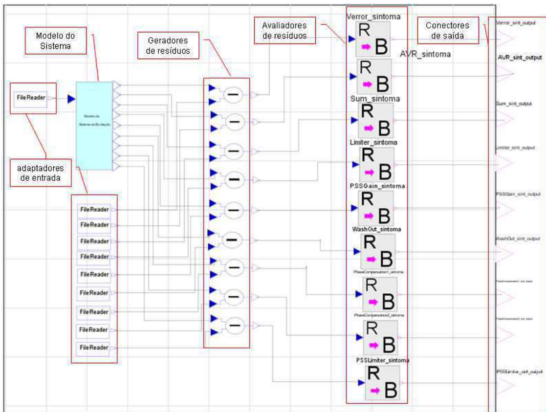
Figura 70: Representação visual do modelo de detecção de falhas
