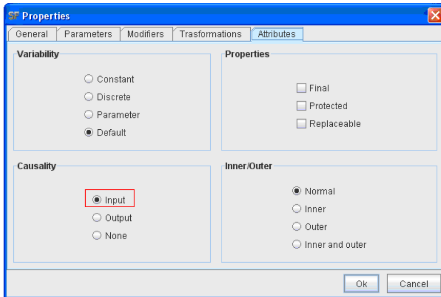
Figura 63: Definindo a causalidade do conector “Verror_input”.
