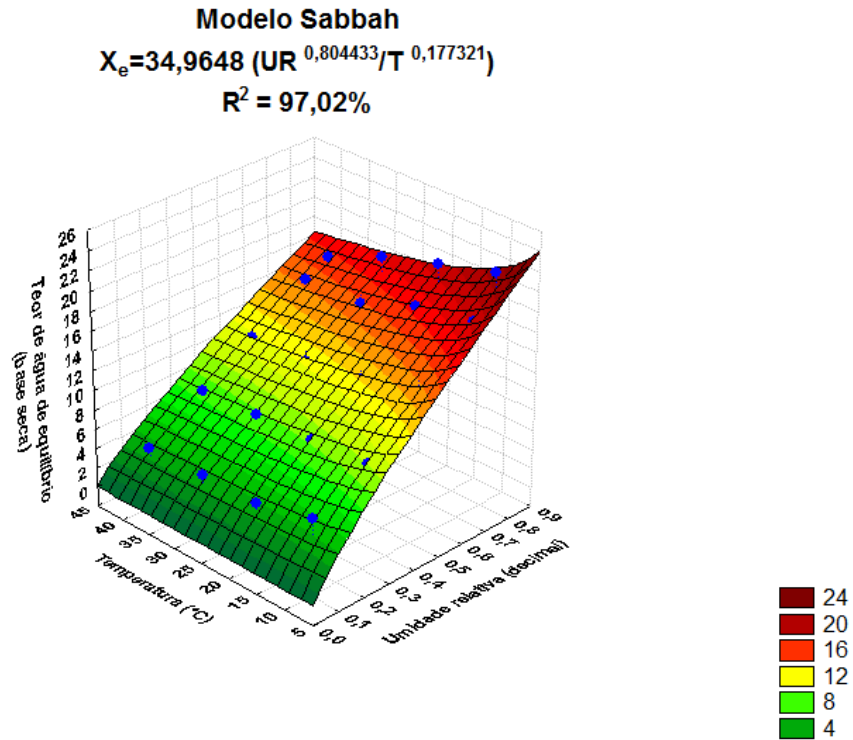
Figura 4.7 - Superfície de resposta das isotermas de dessecção dos grãos de arroz vermelho em casca, estimada pelo modelo de Sabbah, para diferentes condições de temperatura e umidade relativa do ar
