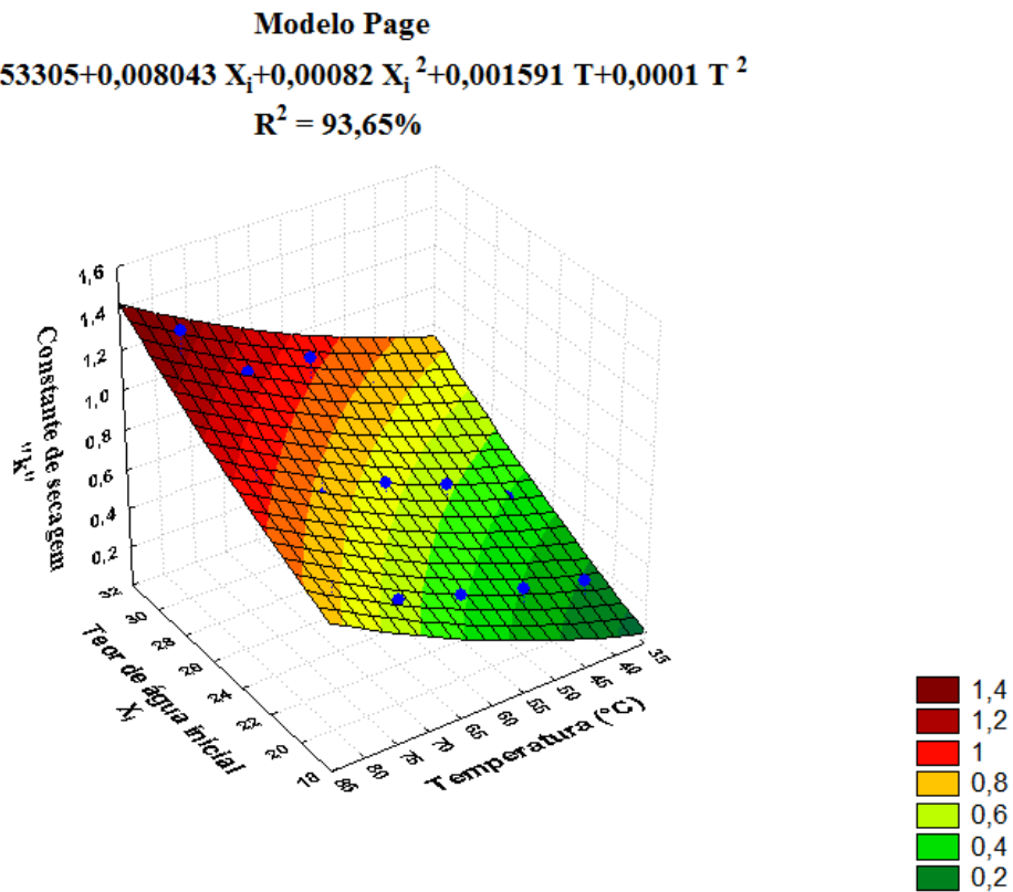
Figura 4.13 – Superfície de resposta do parâmetro “k” da equação de Page em função do teor de água inicial e da temperatura do ar de secagem, obtidos por regressão não linear
