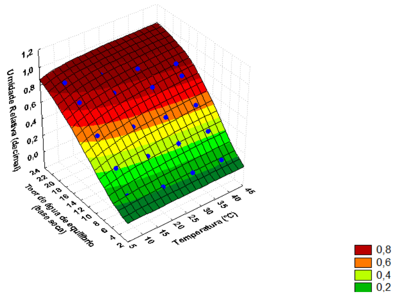
Figura 4.3 - Superfície de resposta das isotermas de dessecção dos grãos de arroz vermelho em casca, estimada pelo modelo de Henderson modificada por Cavalcanti Mata, para diferentes condições de temperatura e umidade relativa do ar
