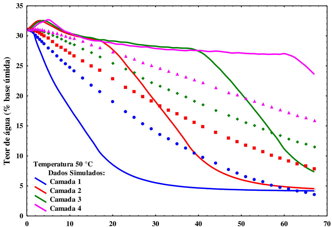
Figura 4.55 - Dados experimentais e simulados da secagem em camada espessa do arroz vermelho em casca com teor de água médio inicial de 30% base úmida e temperatura de 50 °C
