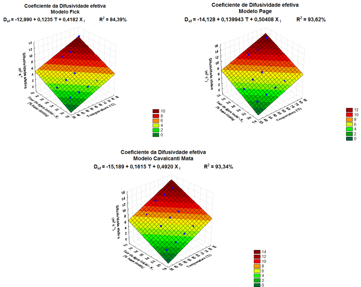
Figura 4.30 - Superfícies de respostas do coeficiente de difusividade efetiva do arroz vermelho em casca, estimada pelos modelos de Fick, Page e Cavalcanti Mata, para diferentes condições de temperatura e teor de água inicial
