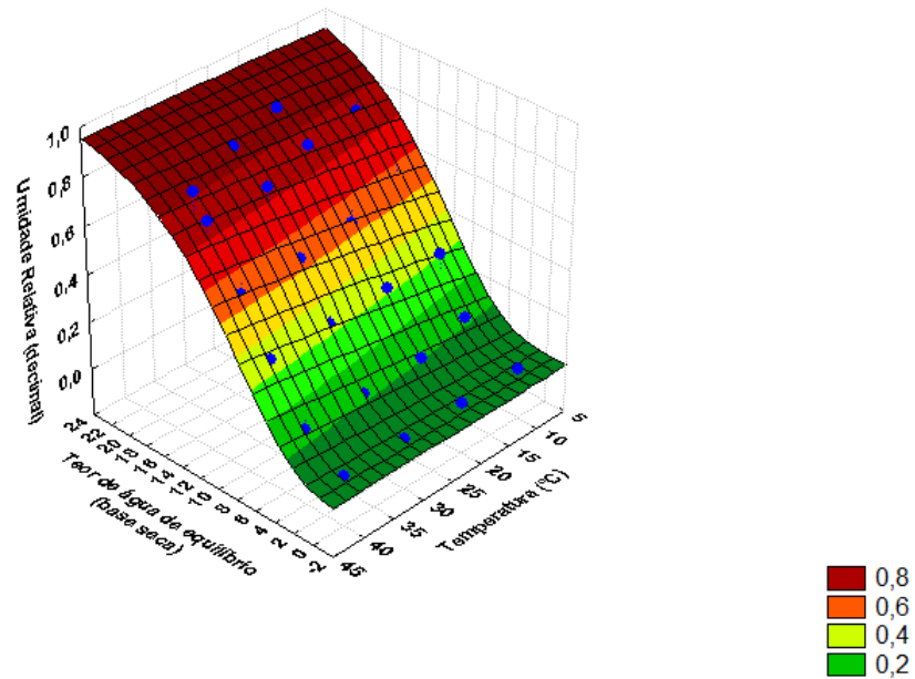
Figura 4.5 - Superfície de resposta das isotermas de desorção dos grãos de arroz vermelho em casca, estimada pelo modelo de Chung-Pfof, para diferentes condições de temperatura e umidade relativa do ar
