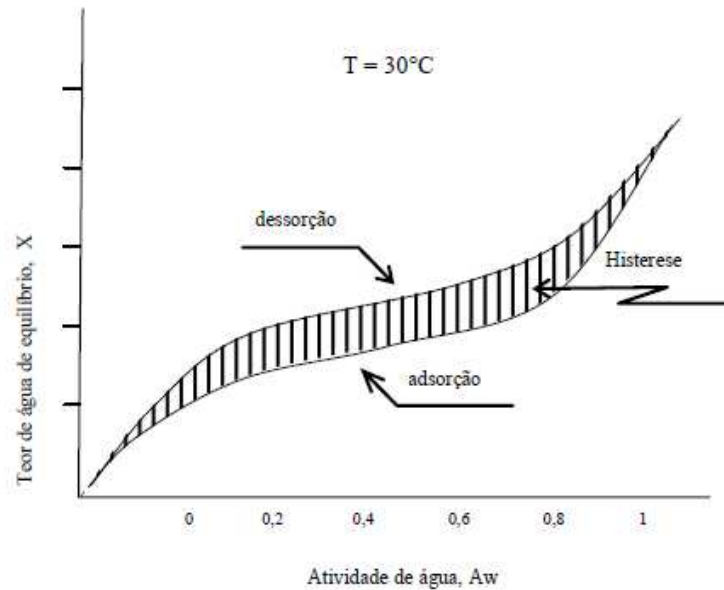
Figura 2.4 - Isotermas de adsorção e dessorção, representação do fenômeno de histerese Fonte: DUARTE, 2006.
