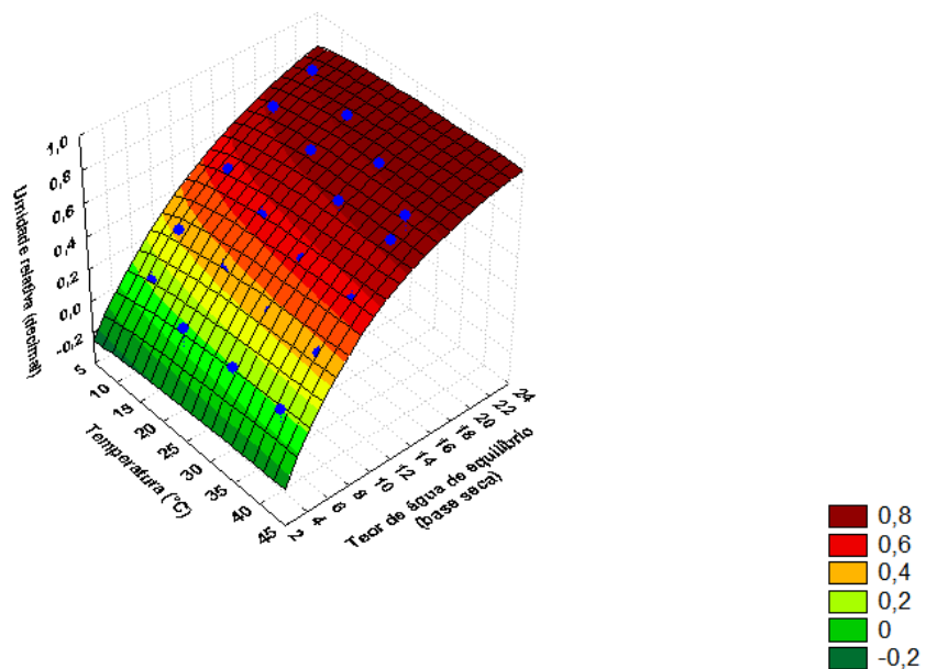
Figura 4.6 - Superfície de resposta das isotermas de desorção dos grãos de arroz vermelho em casca, estimada pelo modelo de Cavalcanti Mata, para diferentes condições de temperatura e umidade relativa do ar
