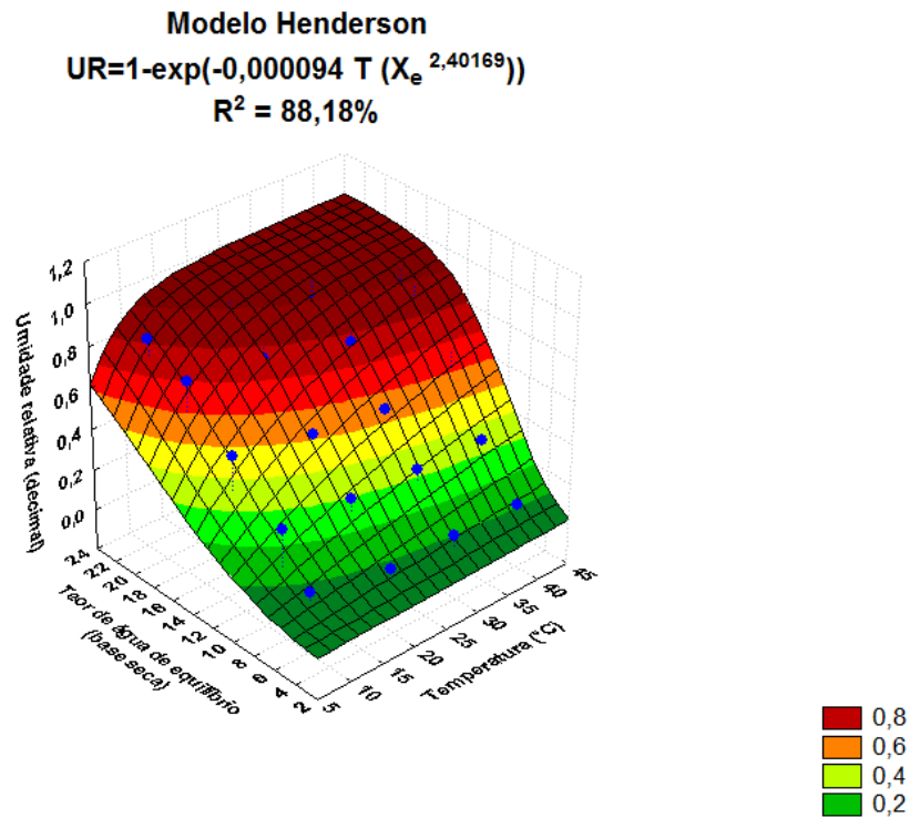
Figura 4.9 - Superfície de resposta das isotermas de dessecção dos grãos de arroz vermelho em casca, estimada pelo modelo de Henderson, para diferentes condições de temperatura e umidade relativa do ar
