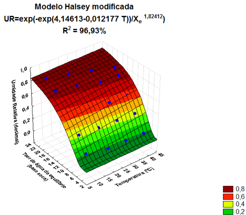
Figura 4.8 - Superfície de resposta das isotermas de dessecção dos grãos de arroz vermelho em casca, estimada pelo modelo de Halsey modificada, para diferentes condições de temperatura e umidade relativa do ar
