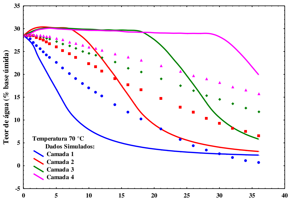
Figura 4.59 - Dados experimentais e simulados da secagem em camada espessa do arroz vermelho em casca com teor de água médio inicial de 30% base úmida e temperatura de 70 °C
