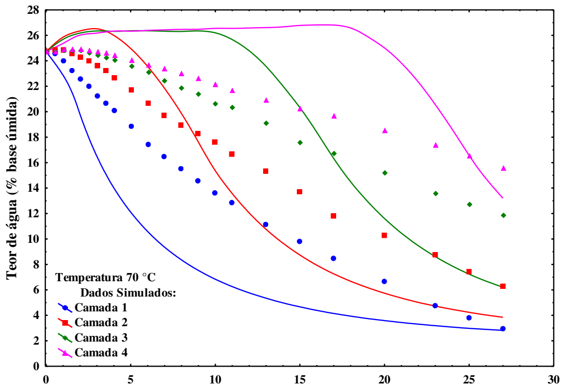
Figura 4.51 - Dados experimentais e simulados da secagem em camada espessa do arroz vermelho em casca com teor de água médio inicial de 25% base úmida e temperatura de 70 °C
